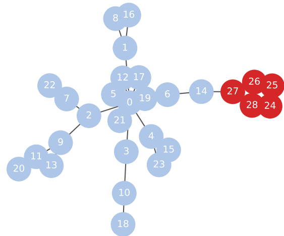
Cycle Motif
