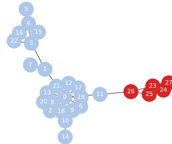
House Motif
