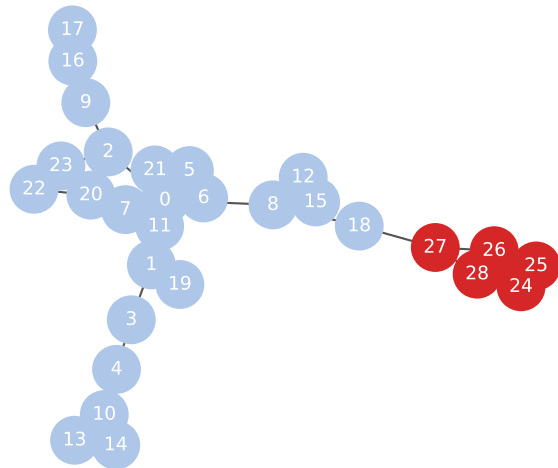
Cycle Motif
