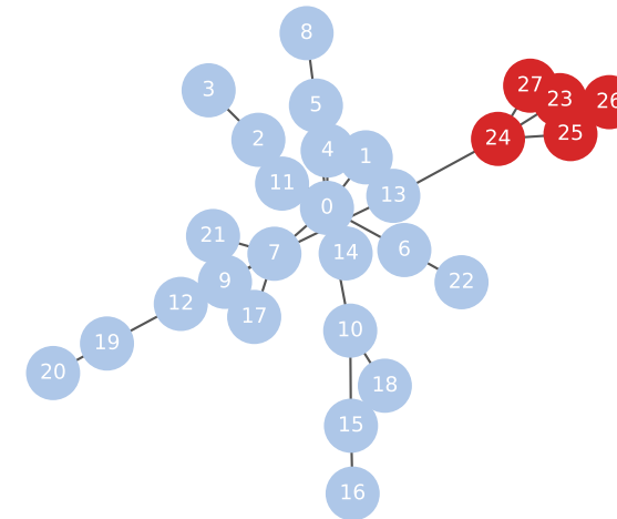
House Motif
