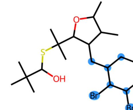
di_bromo_ortho
