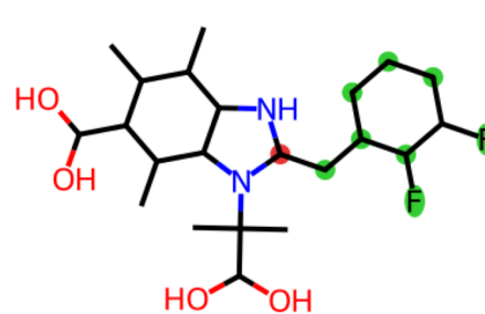
Pred: di_fluoro_ortho
