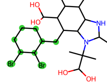
Pred: di_bromo_ortho
