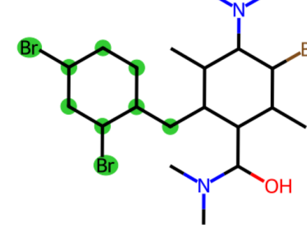
Pred: di_bromo_meta
