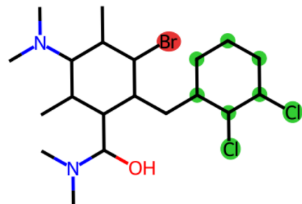
Pred: di_chloro_ortho
