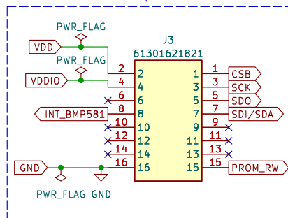
Connecteur d'interface du µC
