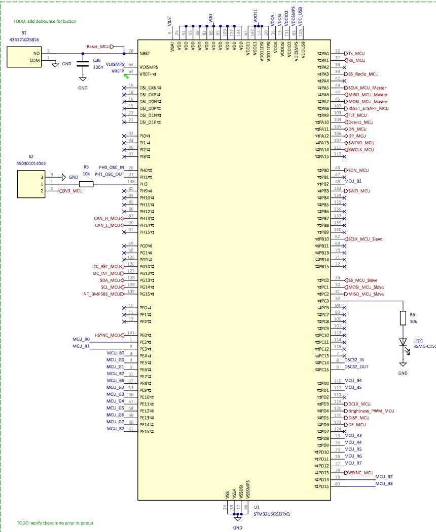
STM32U5G9ZJTxxQ MCU
