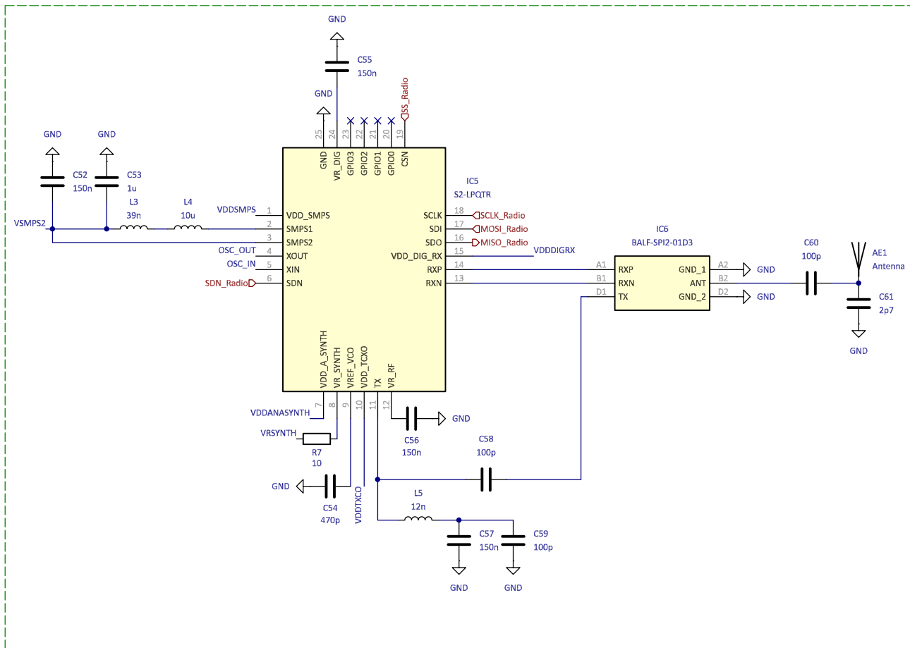
Sub-GHz module
