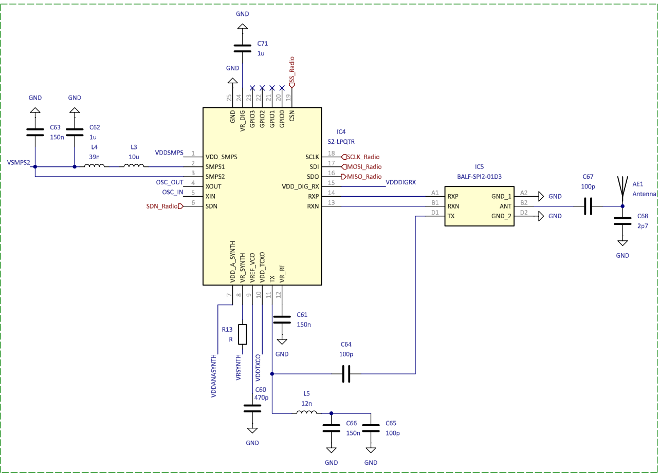
Sub-GHz module
