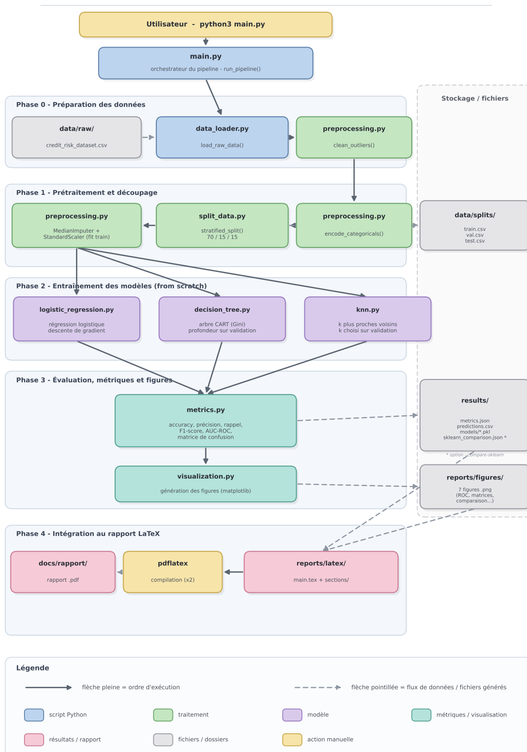
Figure 3 - Schéma d'exécution des scripts du projet : enchaînement du pipeline Python, des données aux modèles, puis aux métriques, figures et rapport.
