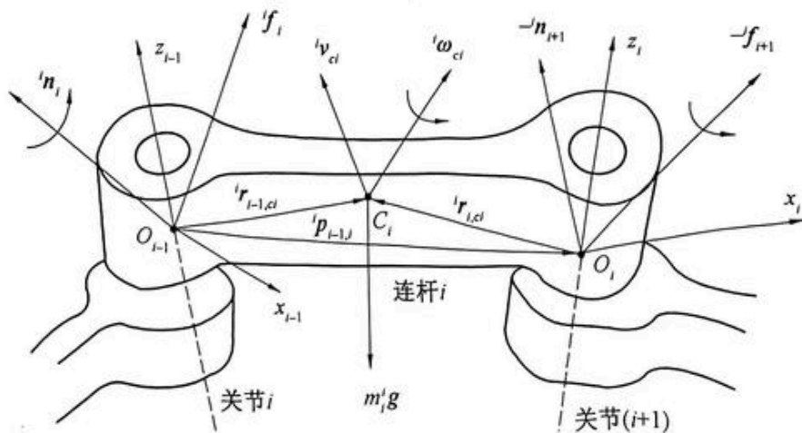
图 10.11 连杆 i 的运动及受力情况
