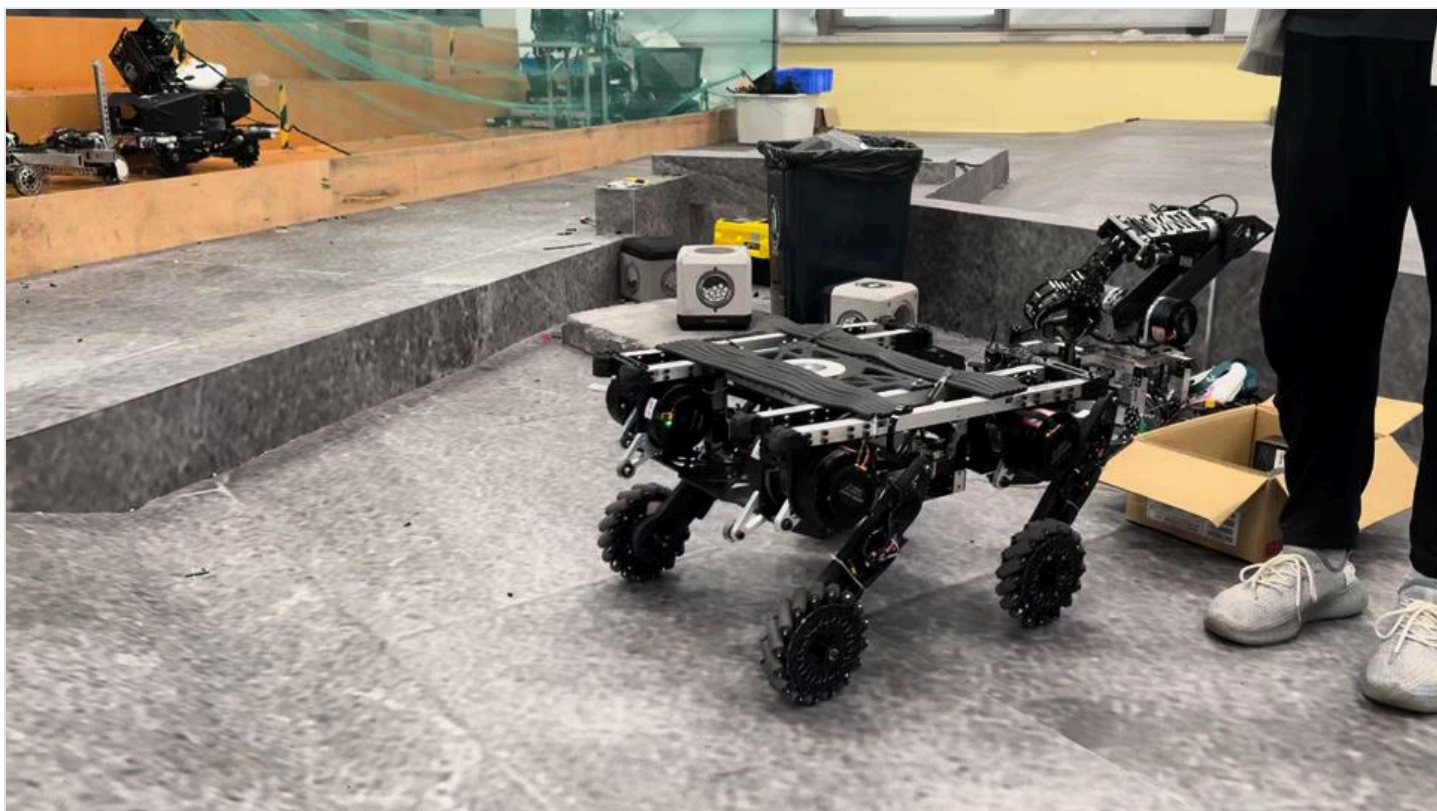
平衡控制效果演示
