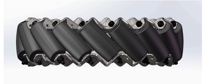
Fig. 3(a). A 型麦克纳姆轮结构。
