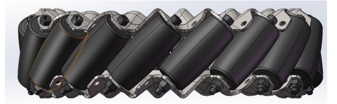
Fig. 3(b). B 型麦克纳姆轮结构。
