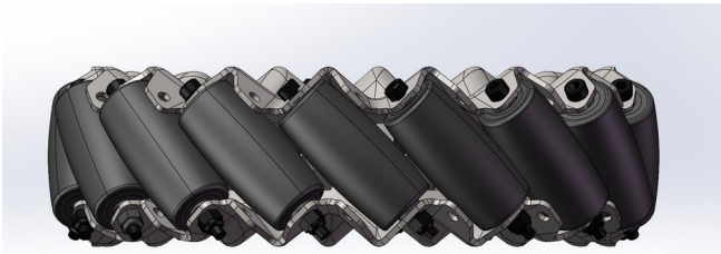
Fig. 3(a). A 型麦克纳姆轮结构。
