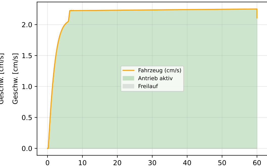
Antrieb & Freilauf
