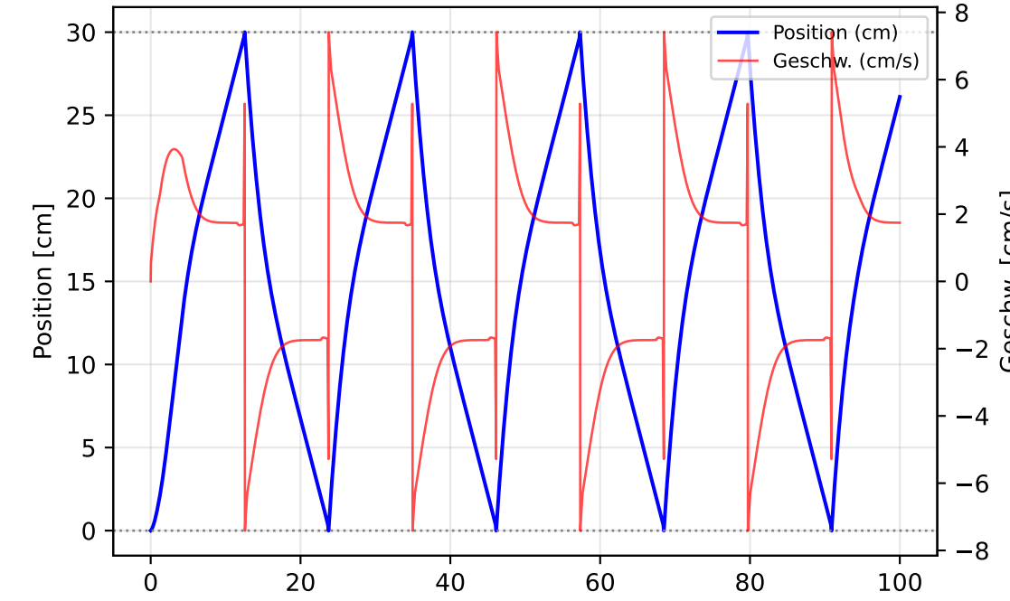
Pneumatik-Zylinder
