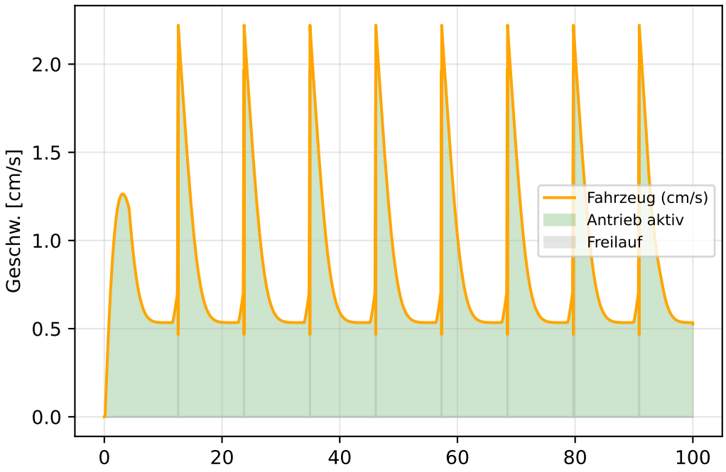
Antrieb & Freilauf
