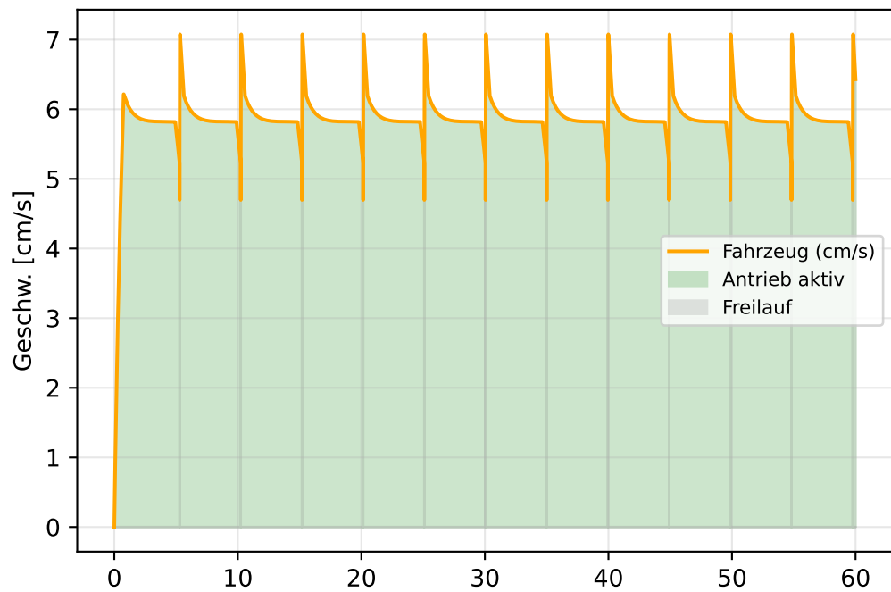
Antrieb & Freilauf
