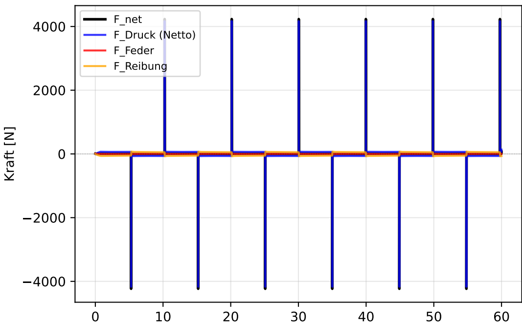
Fahrzeugbewegung
