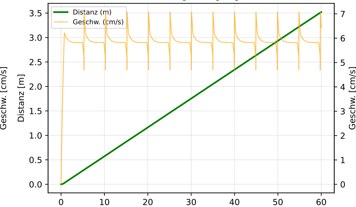
Fahrzeugbewegung
