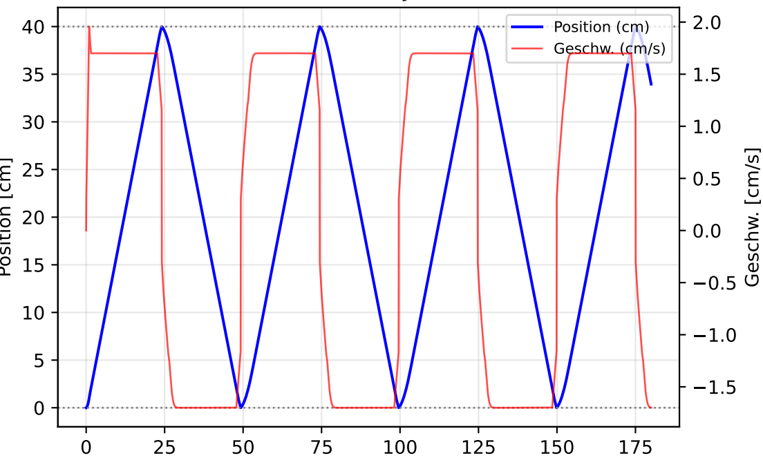
Pneumatik-Zylinder
