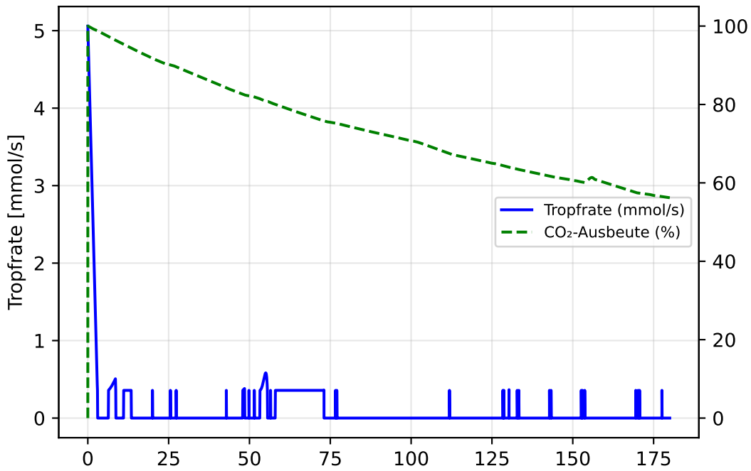
Kolben-Hübe
