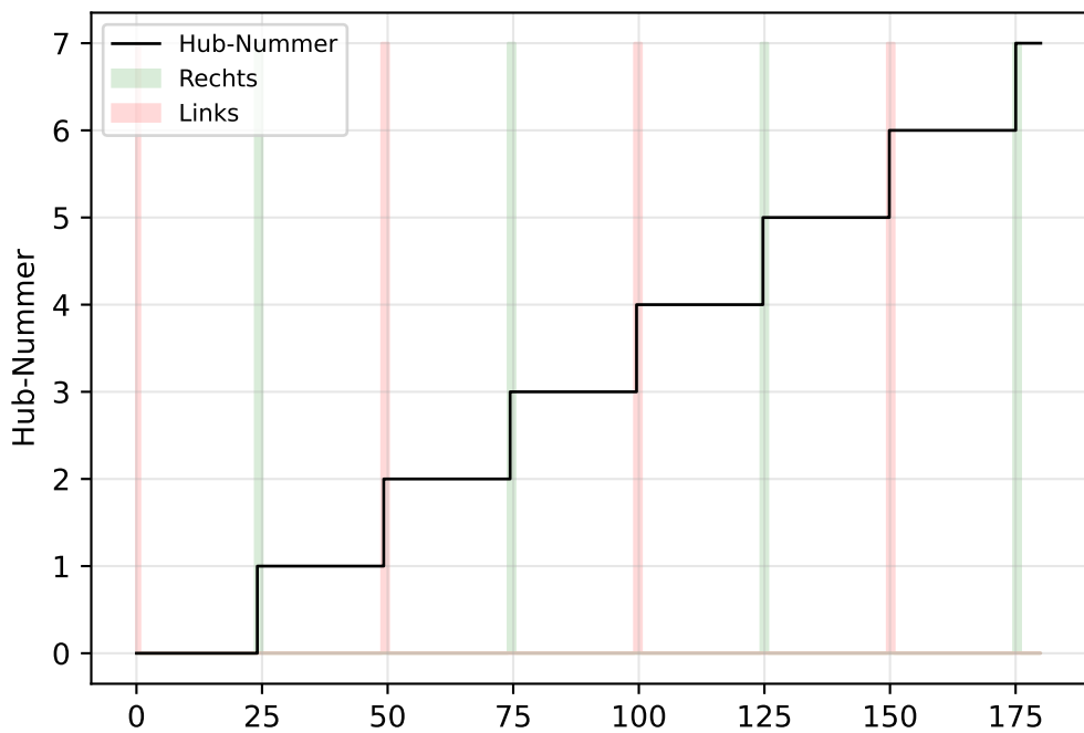
Antrieb & Freilauf
