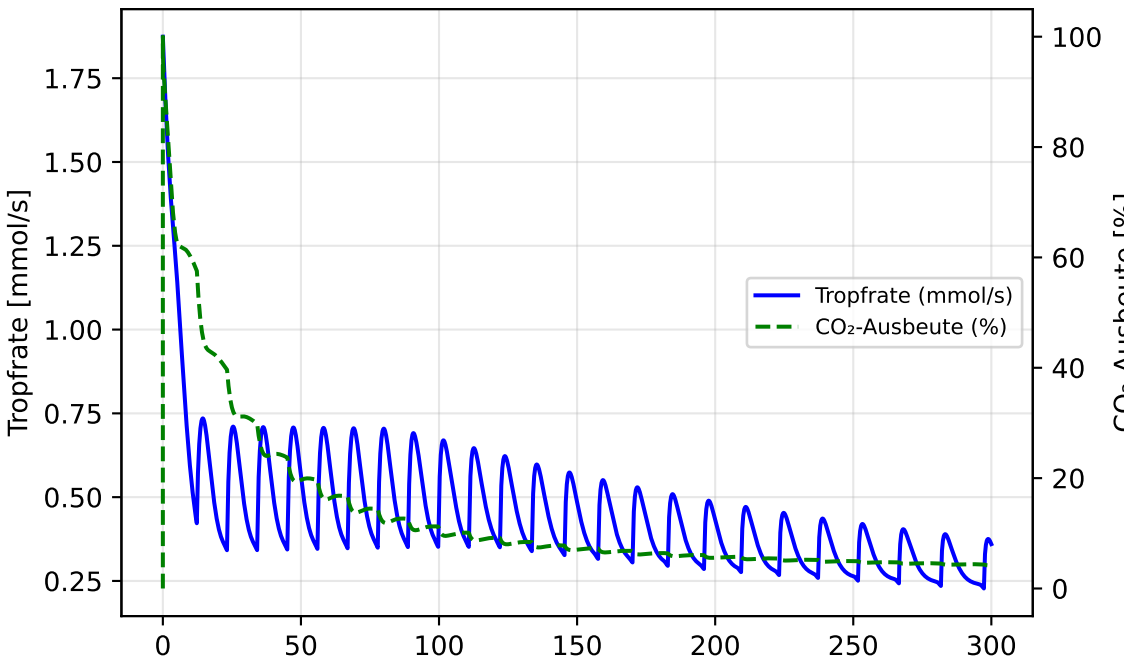
Kolben-Hübe
