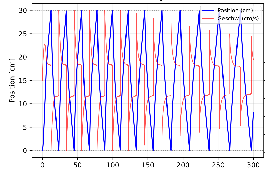
Pneumatik-Zylinder
