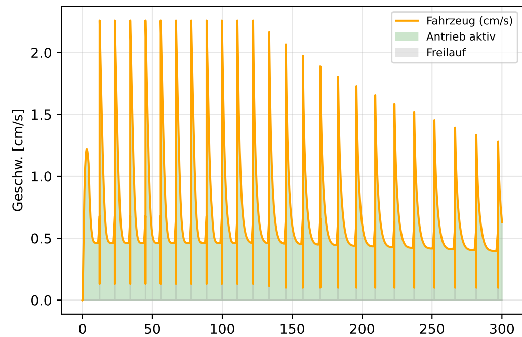
Antrieb & Freilauf
