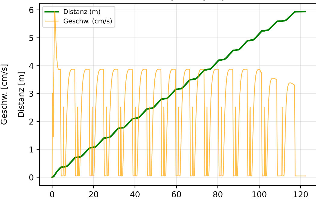
Fahrzeugbewegung
