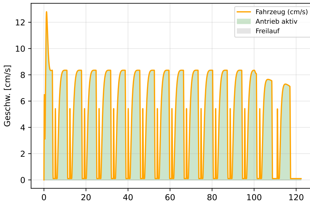
Antrieb & Freilauf
