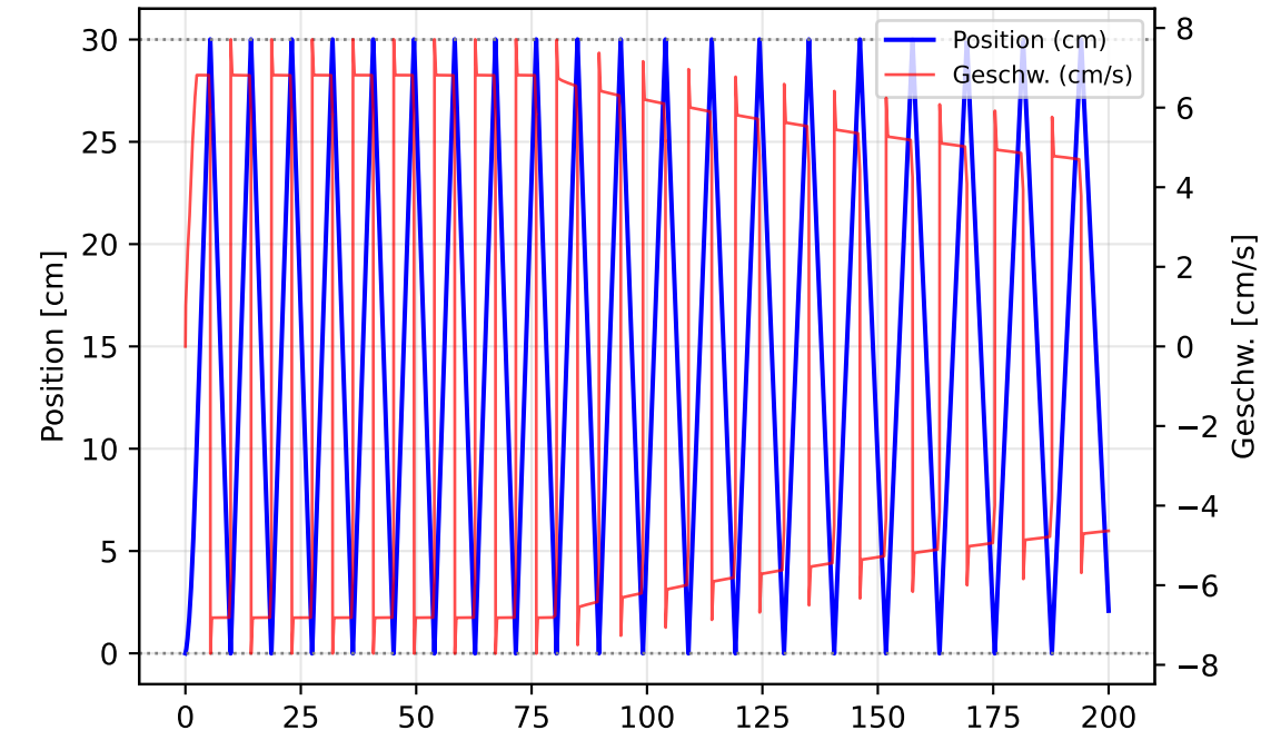
Pneumatik-Zylinder
