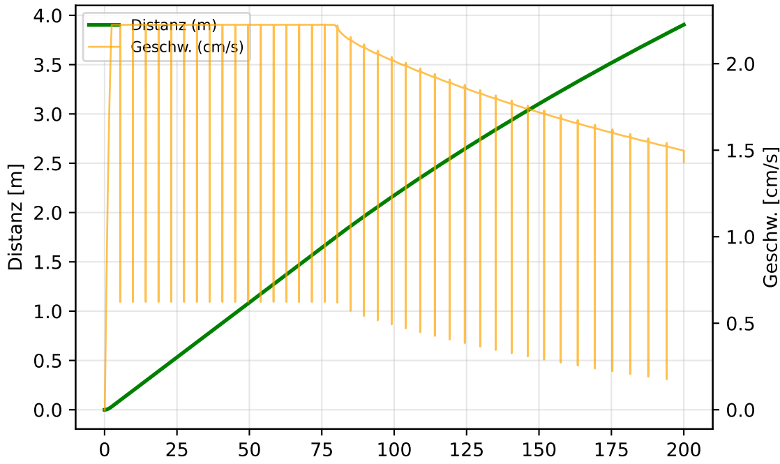
Fahrzeugbewegung
