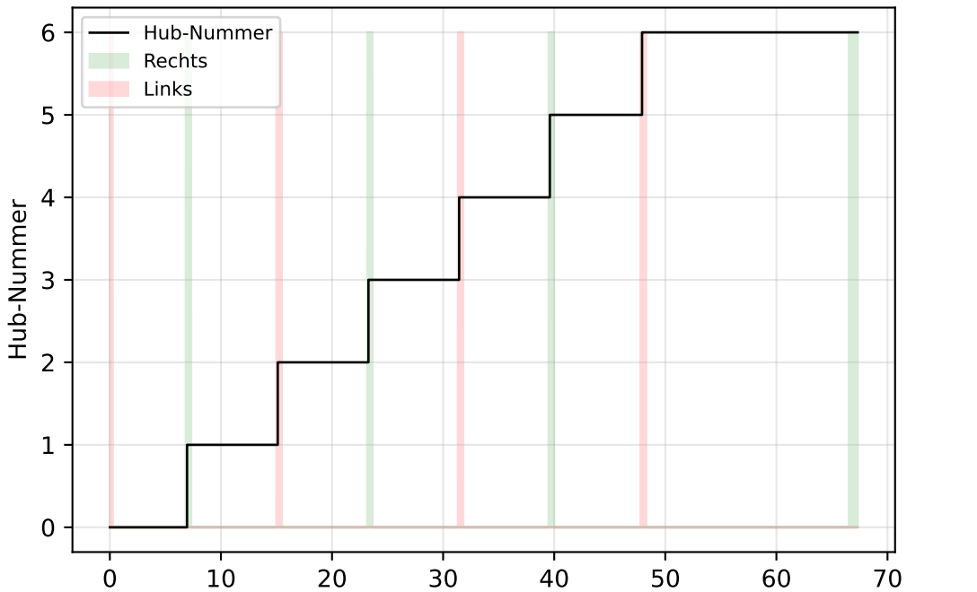
Antrieb & Freilauf
