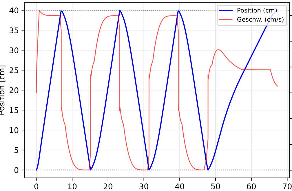
Pneumatik-Zylinder
