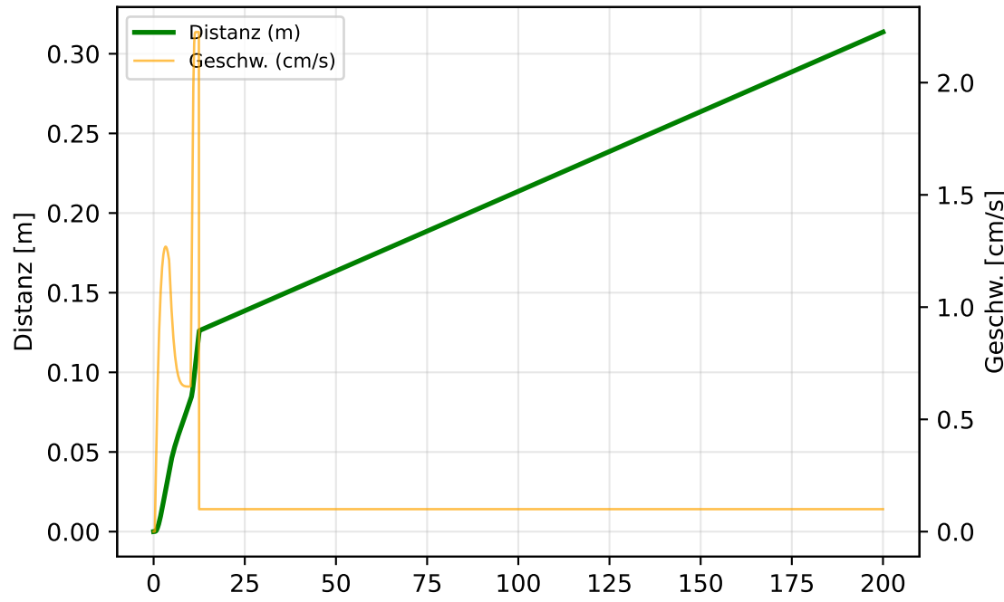
Fahrzeugbewegung
