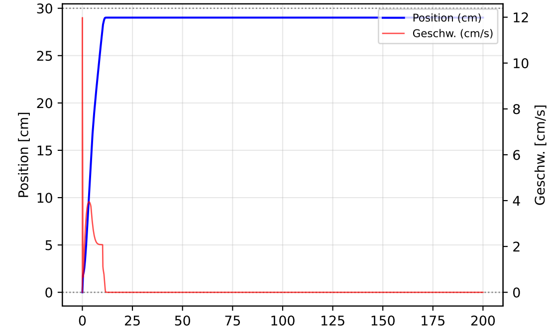
Pneumatik-Zylinder
