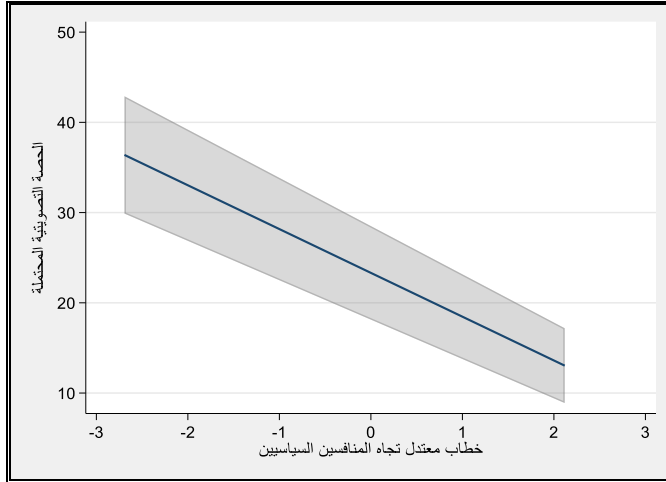
شكل رقم (1): مخطط margins plot
