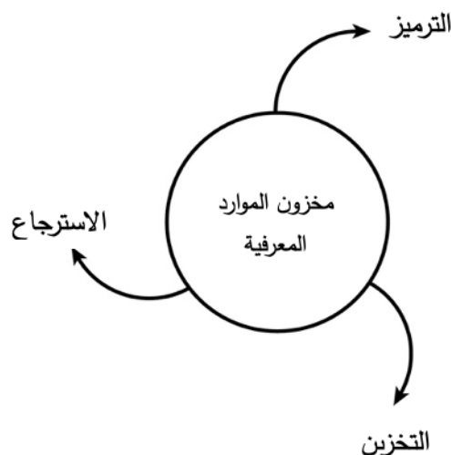
شكل (1) التحديث المفاهيمي المقترح لنموذج LC4MP
