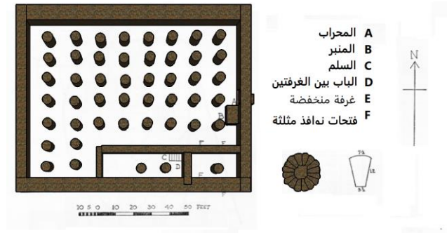
شكل رقم (١٦) مسقط أفقي لمسجد شوبا (عمل الباحث)
