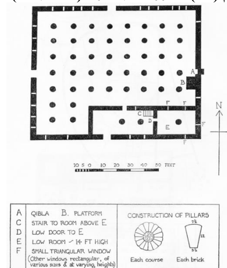
شكل رقم (١٥) مسقط أفقي لمسجد شوبا عن بلفور
