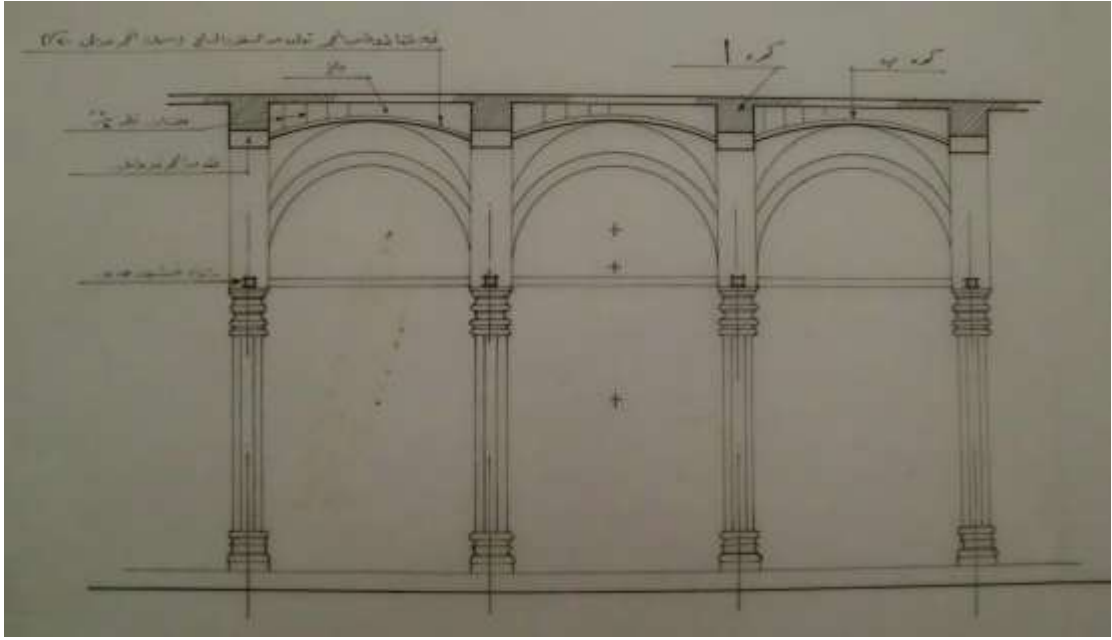
شكل رقم (6): العقود والأعمدة الرخامية لمقعد قايتباي بالحوش السلطاني بالقلعة. عن مركز تسجيل الآثار بالقلعة
