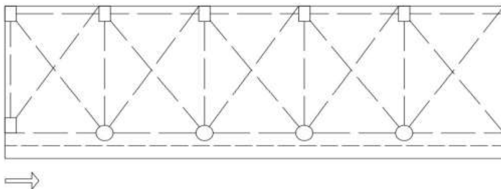
الشكل رقم (4): مسقط أفقي لمقعد السلطان قايتباي بالحوش السلطاني بالقلعة (عمل الباحث)
