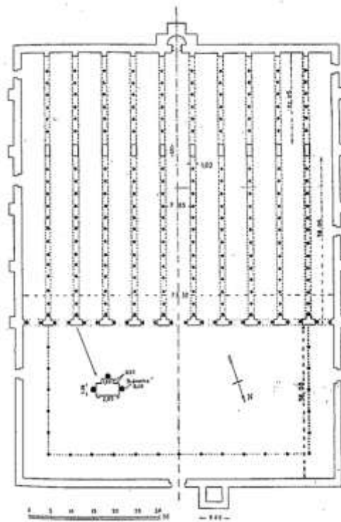
شكل (2): جامع قرطبة، مسقط أفقي، بعد توسعة الأمير عبد الرحمن الأوسط، عن: بالباس. تاريخ إسبانيا الإسلامية. ص496، شكل (187).
