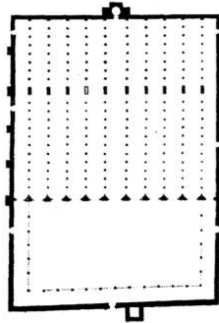
شكل (1): جامع قرطبة، مسقط أفقي، في عهد الأمير عبد الرحمن بن الحكم، عن: مورينو. الفن الإسلامي في إسبانيا. ص54، شكل (47).
