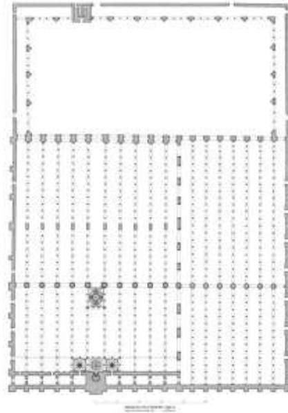
شكل (4): جامع قرطبة، مسقط أفقي، بعد الزيادة العامرية. تصميم المهندس المعماري: "أنطونيو ألماجرو"، عن:
