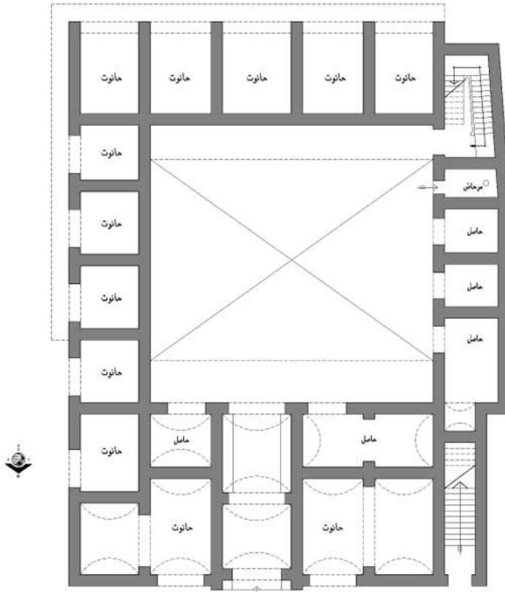
(شكل 1) مخطط تخيلي للطابق الأرضي لوicale أمة الله قادن زوجة ومعتوقة عبد الرحمن كنتخدا من خلال حجة الوقف. بمعرفة الباحث
