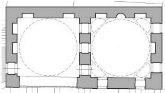
شكل (٢٦) مسقط أفقي لمكتب صبيان مهرماه سلطان باسكودار نقلاً عن Balcan, Mimar Sinan'in
