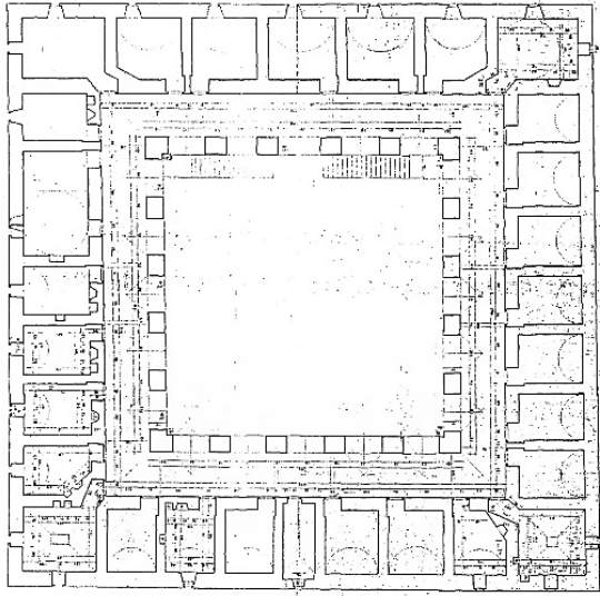
شكل (١٤) مسقط أفقي للطابق الأول لخان قورشونلى Baş, Beylikler Dönemi Hanları, نقلاً عن plan31 a
