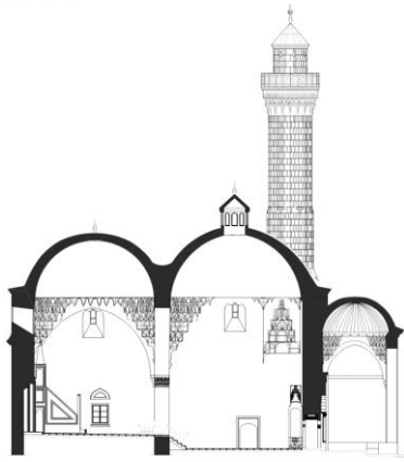
شكل (٨) قطاع رأسى لمسجد كلية إسماعيل بك نقلًا عن Vakıflar Genel Müdürlüğü
