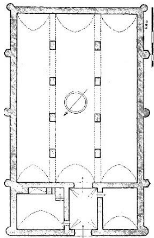
شكل (٣١) مسقط أفقي لخان تاش بقسطنطينية نقلاً عن Baş, Beylikler Dönemi Hanları, plan22
