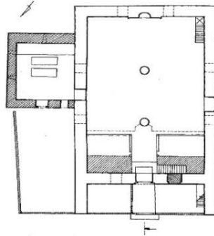
شكل (٢١) مسقط أفقي لمسجد إسماعيل بك إسفنديار او غلو بقرية كورة الحديد بقسطنطينية نقلاً عن Eser, Kûre-i Hadid Köyü'nde Candaroğlu İsmail
