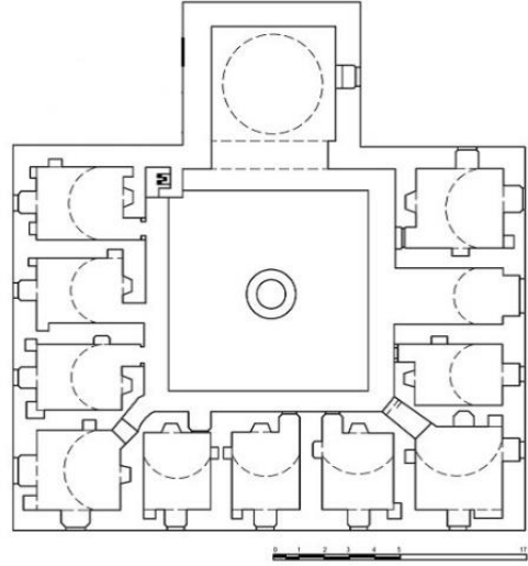
شكل (٩) مسقط أفقي لمدرسة إسماعيل إسفنديار اوغلو بقسطنطينية نقلاً عن Şahin, Morçöl, Kastamonu İsmail Bey Külliyesi Rölövesi
