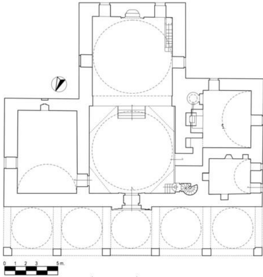
شكل (٤) مسقط أفقي لمسجد كلية إسماعيل بك نقلاً عن Vakıflar Genel Müdürlüğü
