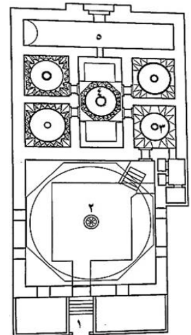
شكل (٣٠) مسقط أفقي لحمام عمر بك Gabriel, Une capitale
