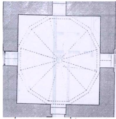
شكل (٢٧) مسقط أفقي لمدرسة صوباشي عيني بك نقلاً عن Ayverdi, Osmanlı mi'mârîsinin ilk devri. شكل (٢٨) مسقط أفقي لتربة أخى شرف الدين بأنقرة نقلاً عن Acun, İnci, Ankara Ahi şerafettin Zaviyesi (نقلاً عن Ayverdi, Osmanlı mi'mârîsinin ilk devri). شكل (٢٩) مسقط أفقي حمام كلية السلطان مراد الثاني (نقلاً عن Ayverdi, Osmanlı mi'mârîsinin ilk devri).
