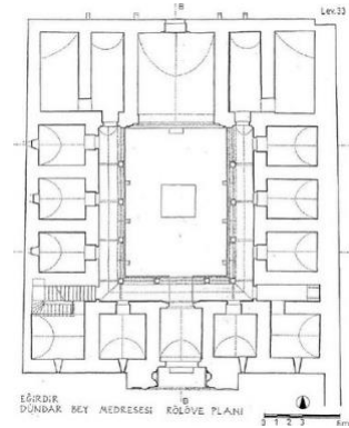
شكل (٢٣) مسقط أفقي لمدرسة دُندار بك نقلاً عن Kuran, Medreseleri
