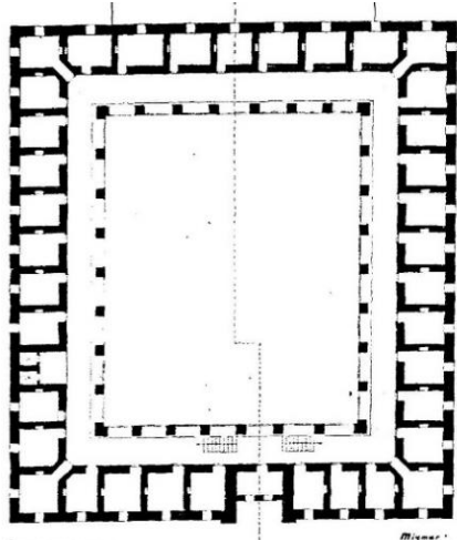
شكل (٣٢) مسقط أفقي للطابق الأرضي لخان الأمير بقسطنطينية نقلاً عن Baş, Beylikler Dönemi Hanları
