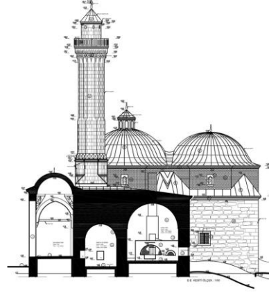
شكل (٧) قطاع رأسى مع واجهة لمسجد كلية إسماعيل بك نقلًا عن Serin, Selçuklu ve Beylikler Dönemi
