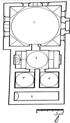
شكل (٢٧) مسقط أفقي لمدرسة صوباشي عيني بك نقلاً عن Ayverdi, Osmanlı mi'mârîsinin ilk devri. شكل (٢٨) مسقط أفقي لتربة أخى شرف الدين بأنقرة نقلاً عن Acun, İnci, Ankara Ahi şerafettin Zaviyesi (نقلاً عن Ayverdi, Osmanlı mi'mârîsinin ilk devri). شكل (٢٩) مسقط أفقي حمام كلية السلطان مراد الثاني (نقلاً عن Ayverdi, Osmanlı mi'mârîsinin ilk devri).
