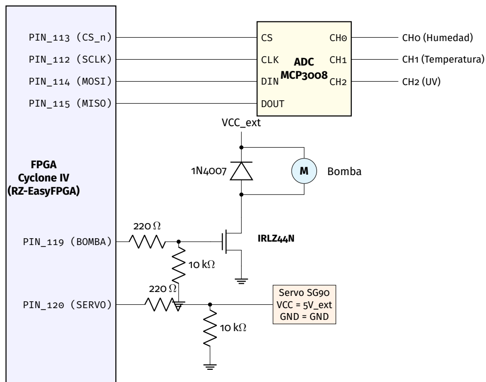
Figura 1: Diagrama de Conexiones Eléctricas del Sistema de Riego.
