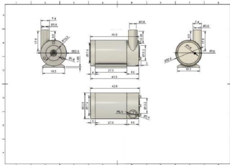
Dimensiones Bomba de Agua Sumergible
