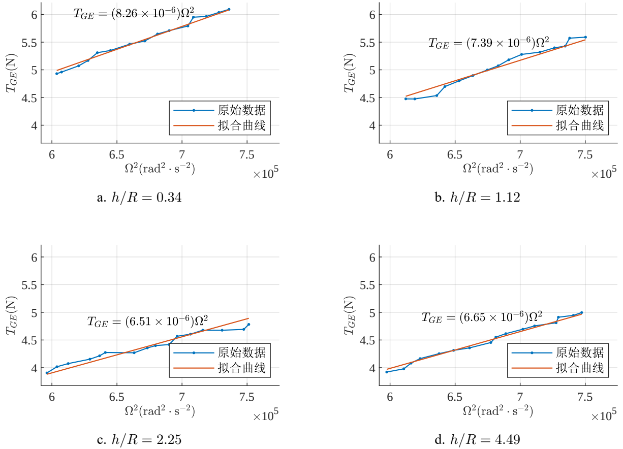
图 4-4 不同高度比 h/R 下推力 T 与风扇转速的平方 \Omega^2 的关系
