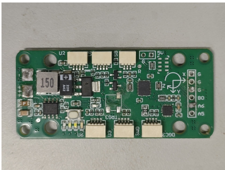
图 2-6 飞行控制板
