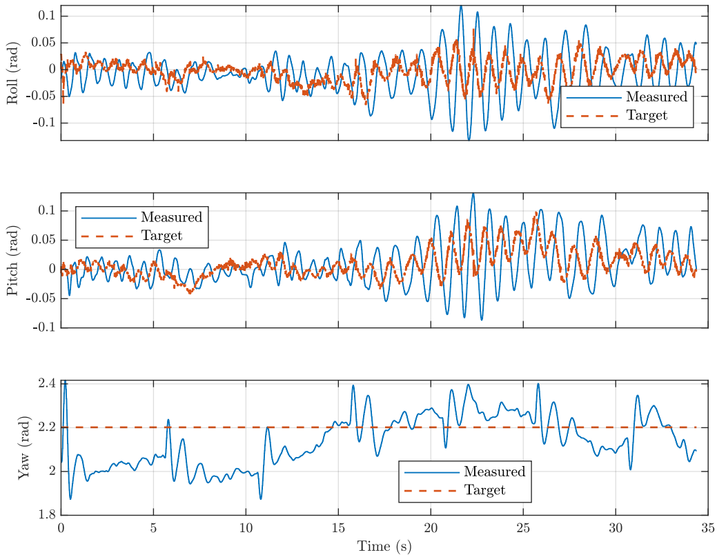
图 5-17 实飞过程中姿态角跟随曲线
