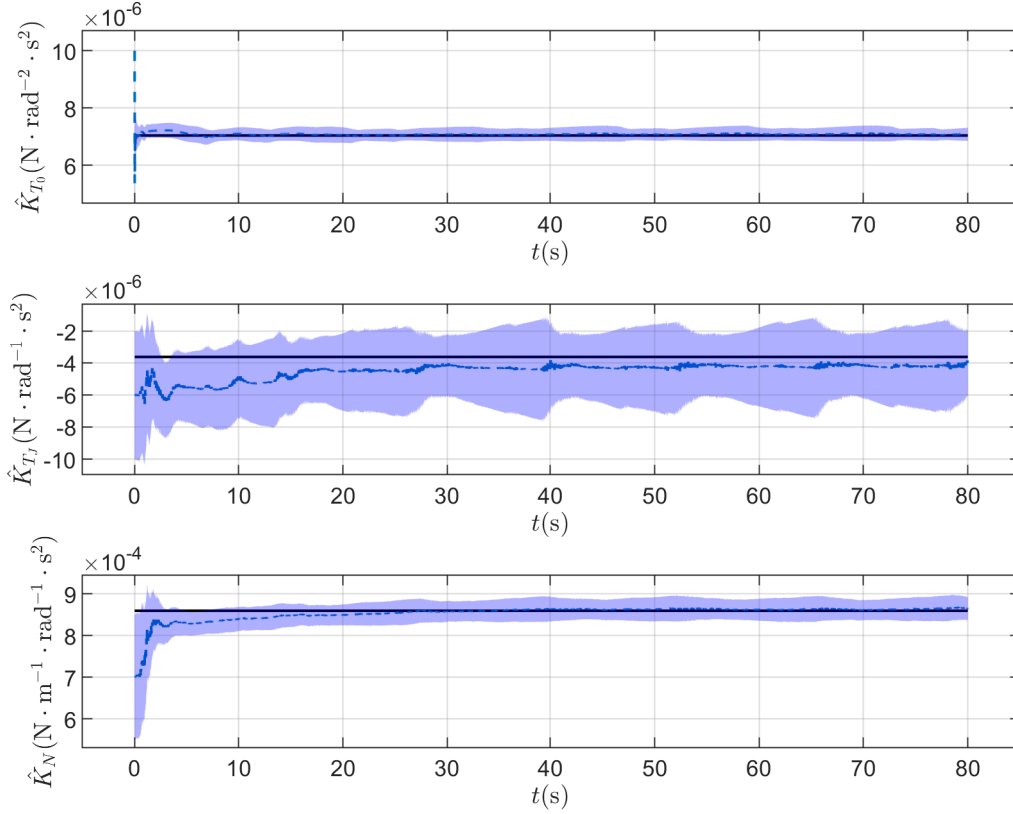
图 3-1 仿真实验气动参数估计结果（一）
