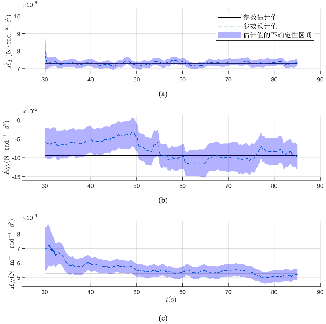
图 3-3 实际飞行试验参数估计结果（一）
