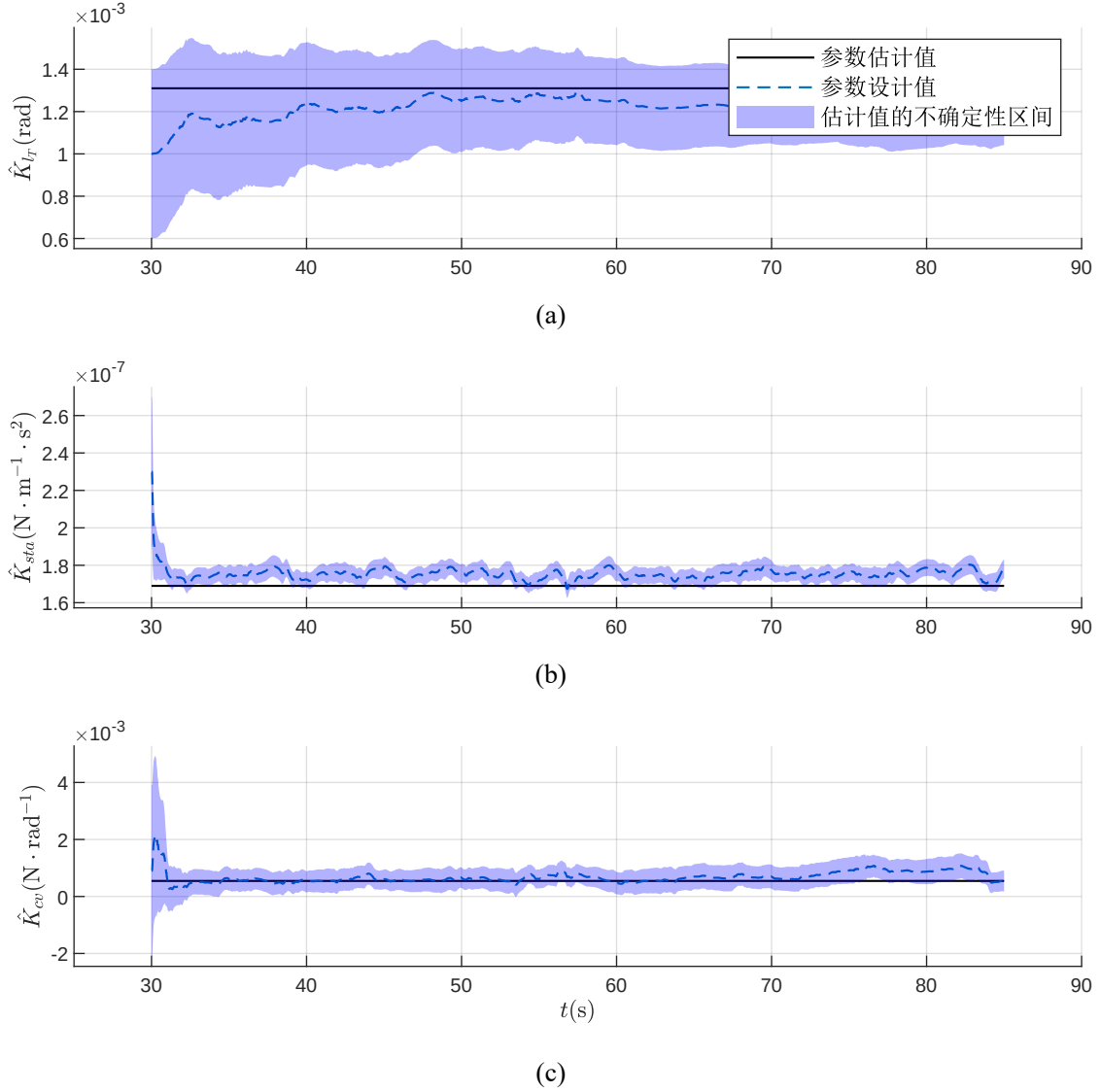
图 3-4 实际飞行试验参数估计结果（二）
