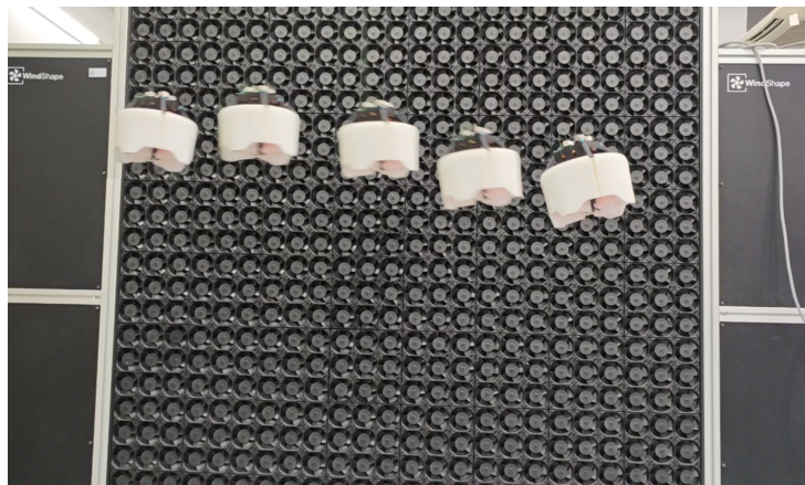
图 3-2 无人机实际飞行试验
