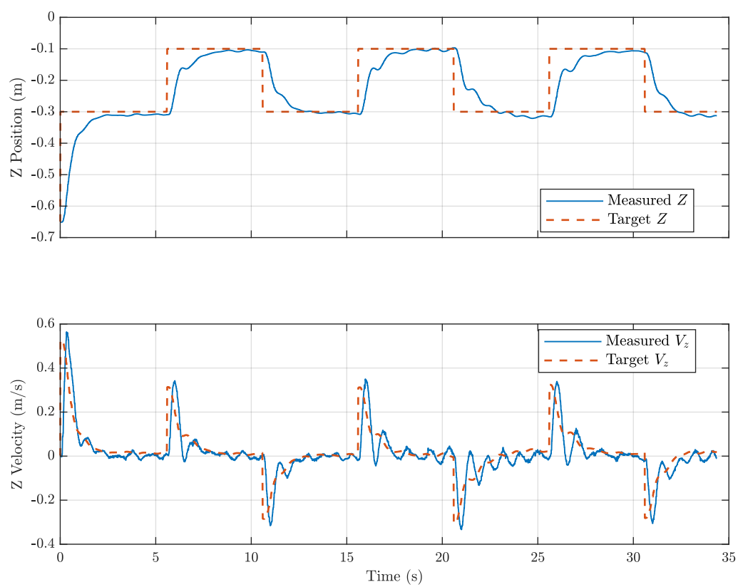
图 5-18 位置速度跟随曲线
