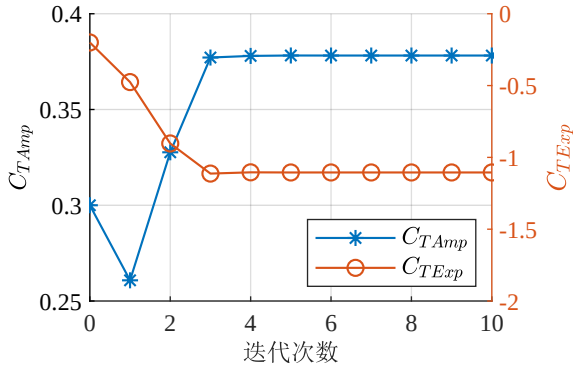
图 4-6 拟合参数与迭代次数的关系
