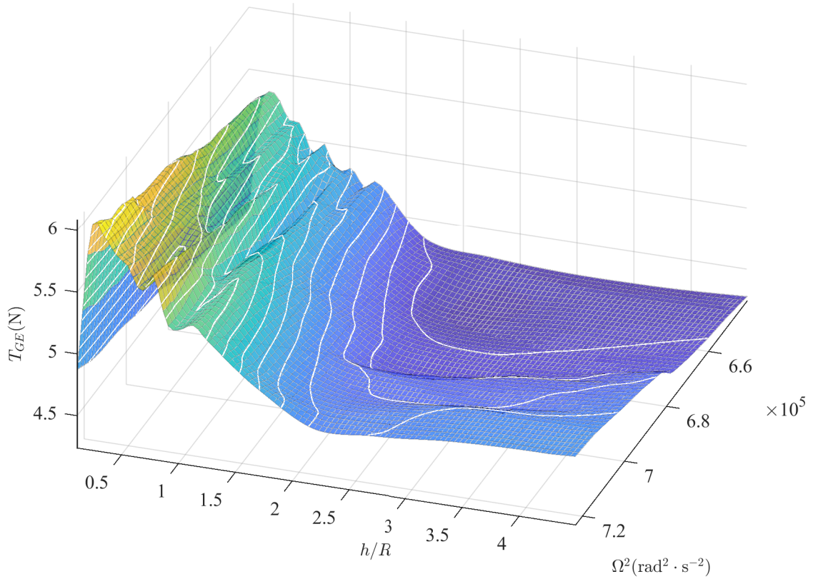
图 4-3 涵道风扇推力和风扇转速、离地高度之间的关系
