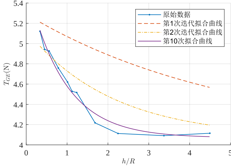
图 4-5 典型工作转速下涵道风扇推力 T 和离地高度比 h/R 的关系
