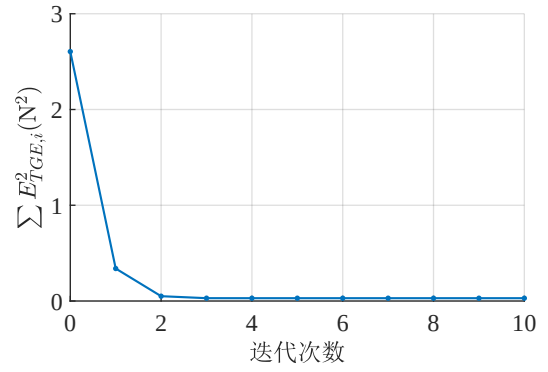
图 4-7 拟合误差平方和与迭代次数的关系
