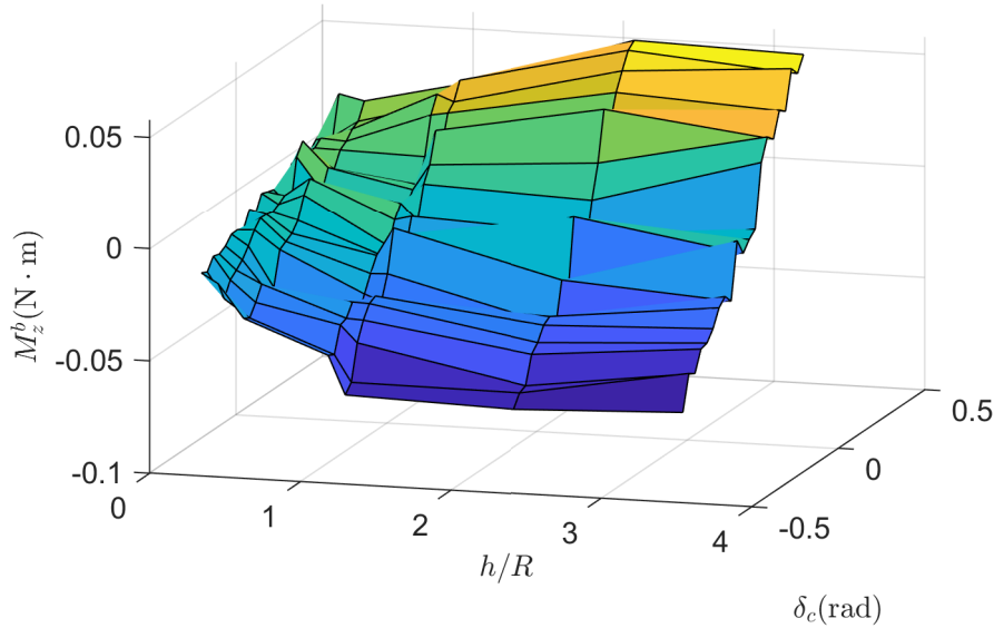
图 4-8 气动力矩 M_z^b 与高度比 h/R 以及控制舵面偏转角度 \delta_c 之间的关系
