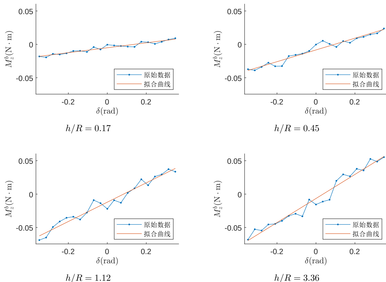
图 4-9 不同高度比 h/R 下扭矩 M_z^b 与舵面角度 \delta 的关系
