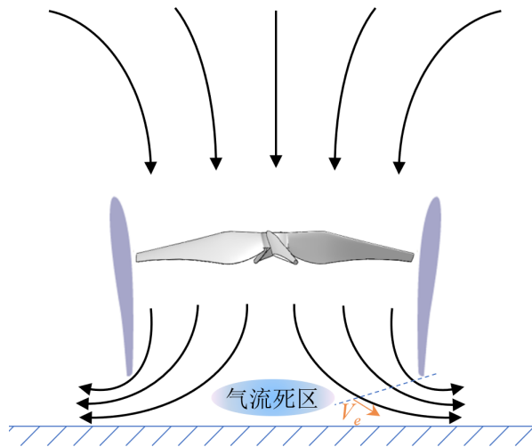
图 4-1 地面效应下气体流动示意图
