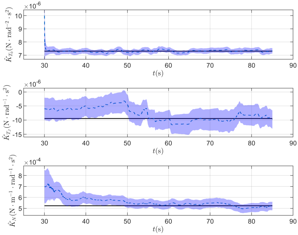
图 3-4 实飞实验气动参数估计结果（一）
