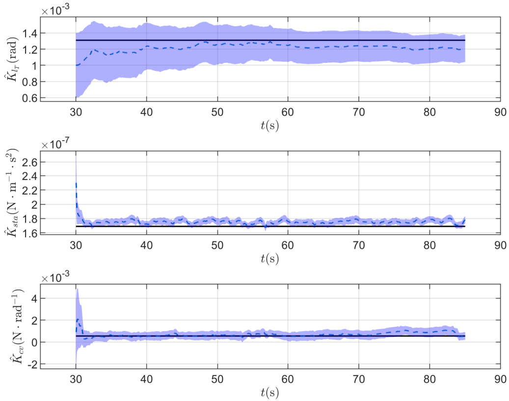
图 3-5 实飞实验气动参数估计结果（二）
