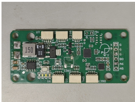
图 2-6 飞行控制板
