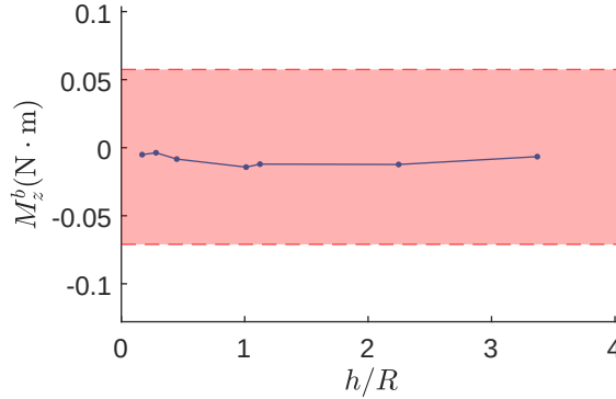
图 4-10 零输出时扭矩 M_z^b 与离地高度 h 的关系
