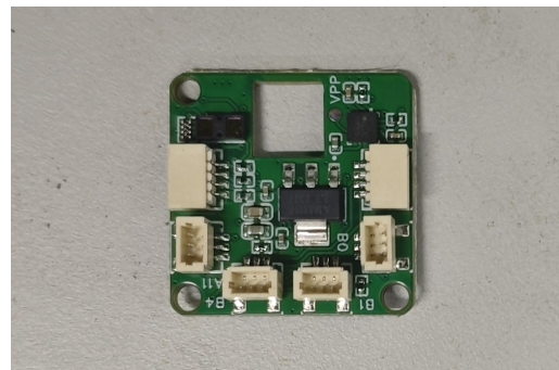
图 2-7 舵机驱动板
