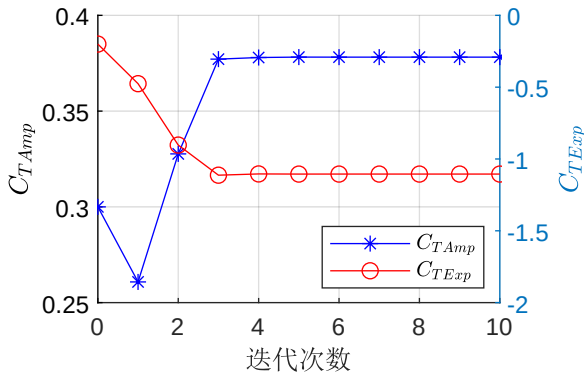
图 4-6 拟合参数与迭代次数的关系
