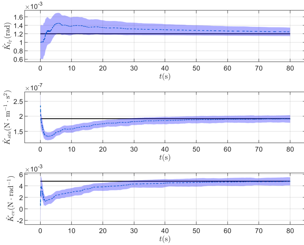
图 3-2 仿真实验气动参数估计结果（二）
