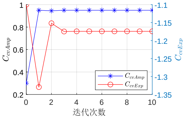
图 4-12 拟合参数与迭代次数的关系
