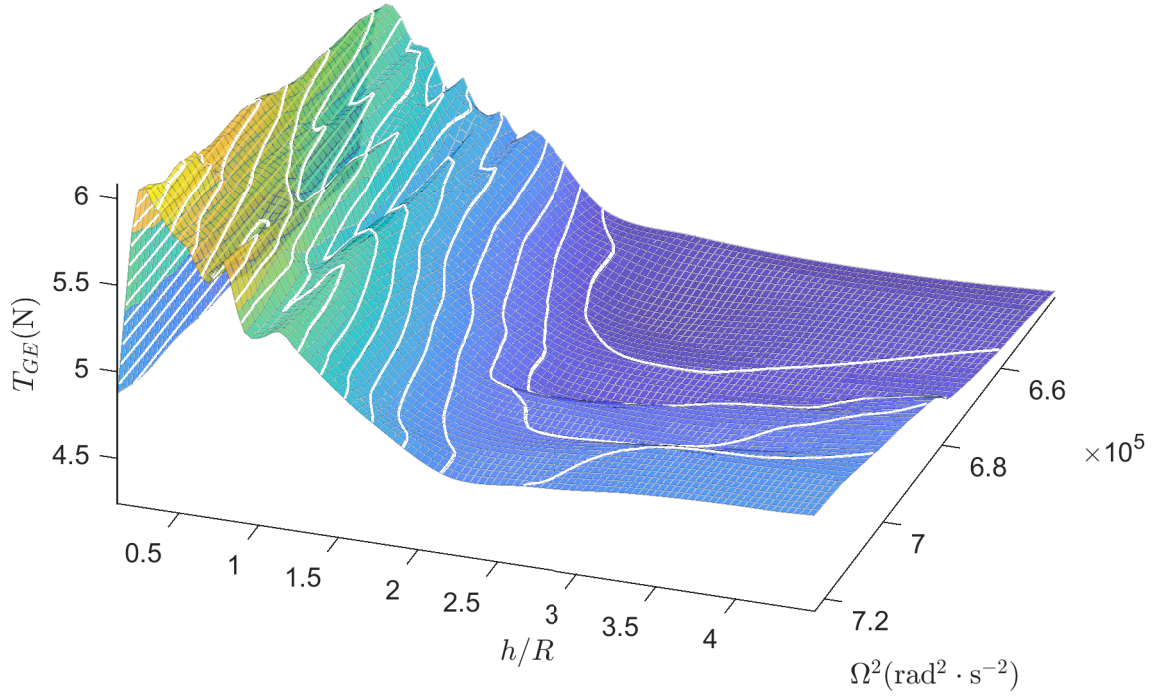
图 4-3 涵道风扇推力和风扇转速、离地高度之间的关系
