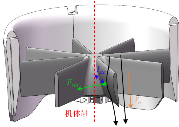
图 2-13 反扭距襟翼作用示意图
