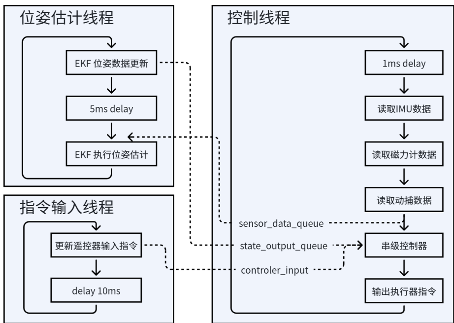
图 2-9 程序设计框图
