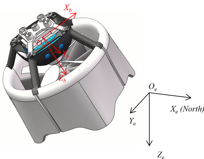
图 2-10 地面坐标系和机体坐标系
