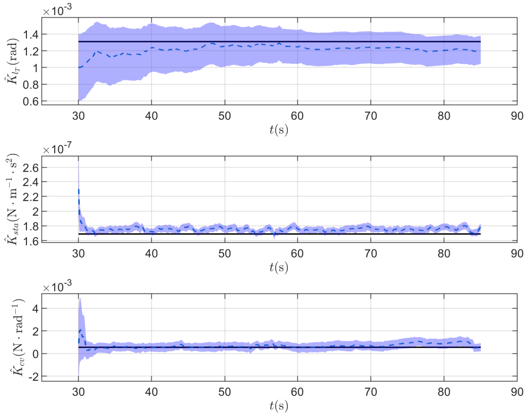
图 3-4 实际飞行试验气动参数估计结果（二）
