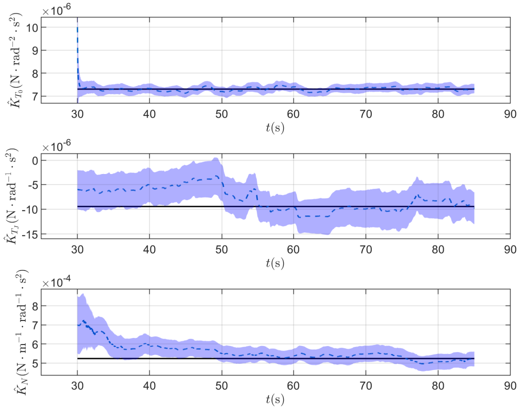
图 3-3 实际飞行试验气动参数估计结果（一）
