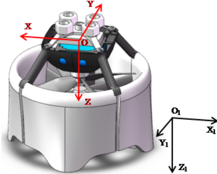
图 2-9 “ZYX 欧拉角”的定义
