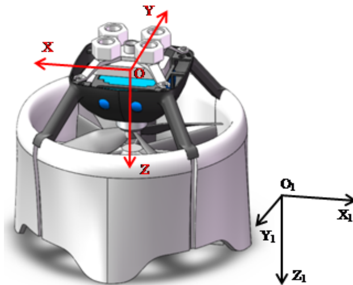
图 2-11 轴流状态的气动分析
