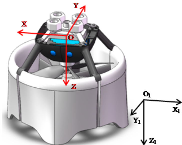
图 2-8 地面坐标系和机体坐标系
