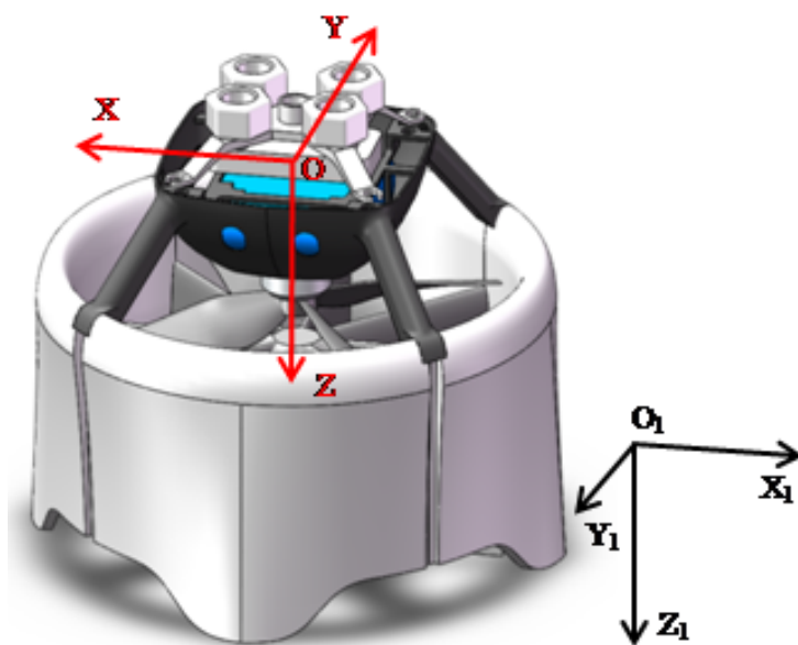
图 2-1 机体结构
