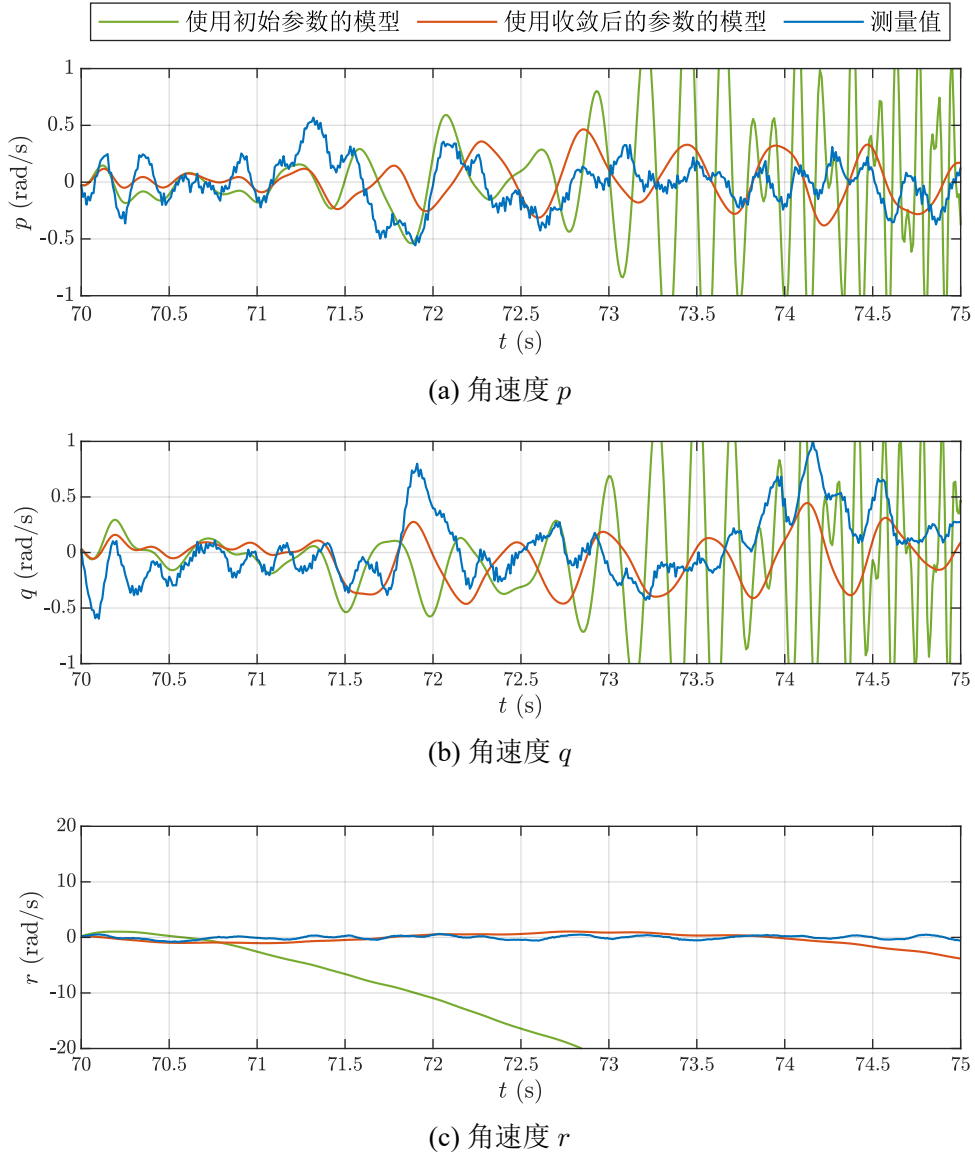
图 3-6 真实飞行角速度与两种模型仿真角速度的对比曲线
