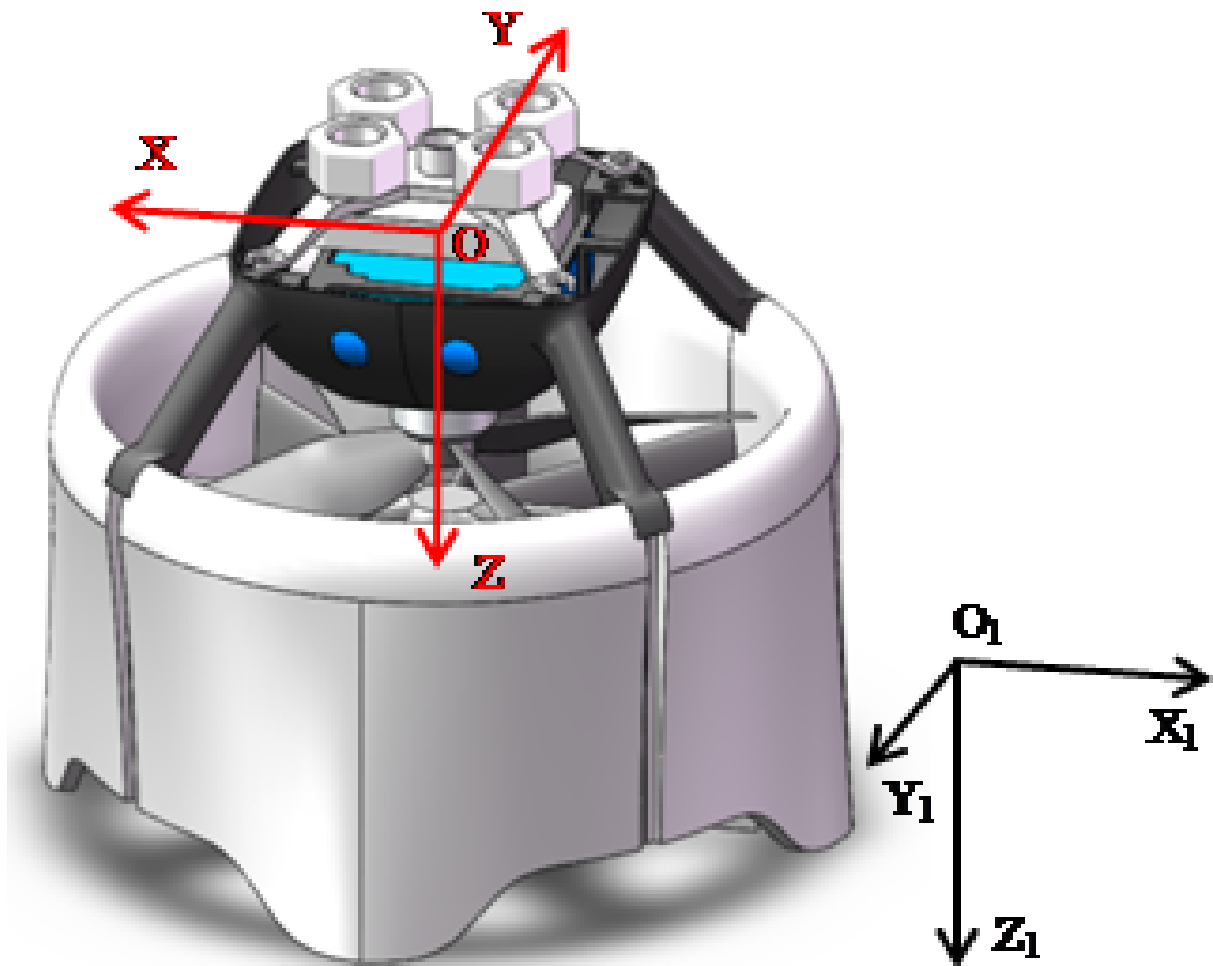
图 2-1 涵道式无人机结构图
