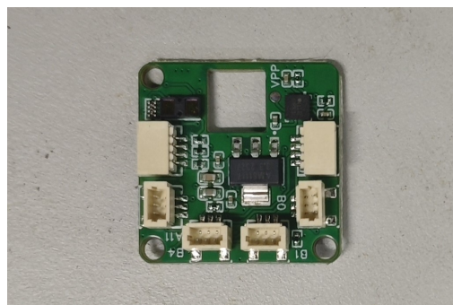
图 2-7 舵机驱动板
