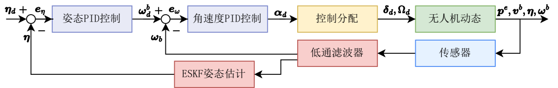
图 5-1 姿态 PID 闭环控制系统框图
