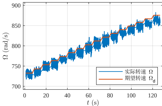
图 5-3 实际转速与期望转速的跟随曲线
