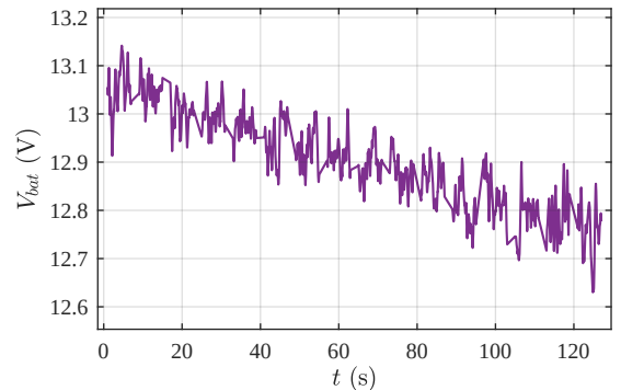
图 5-4 实验过程电压波动曲线
