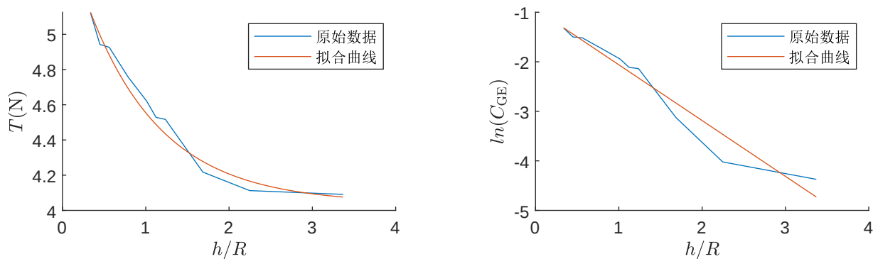
图 4-5 涵道风扇推力和离地高度的关系
