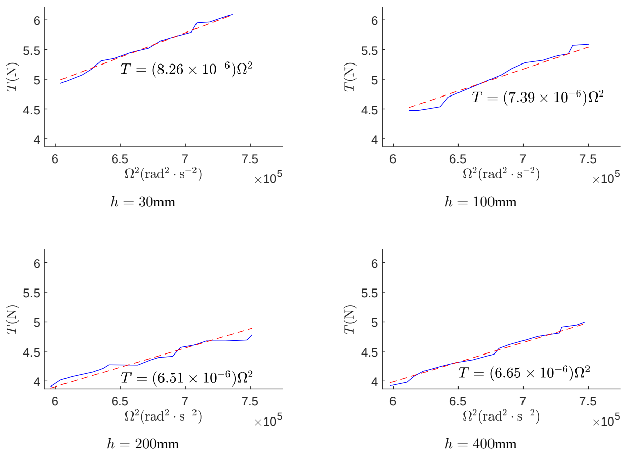
图 4-4 不同高度 h 下推力 T 与风扇转速 \Omega 的关系
