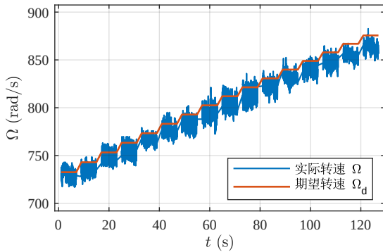
图 5-3 实际转速与期望转速的跟踪曲线
