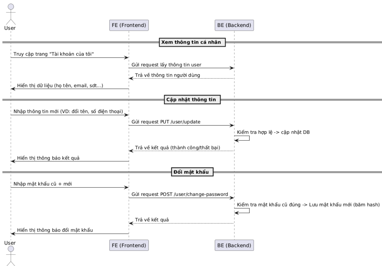
Hình 10 Sơ đồ tuần tự quản lý trang cá nhân
