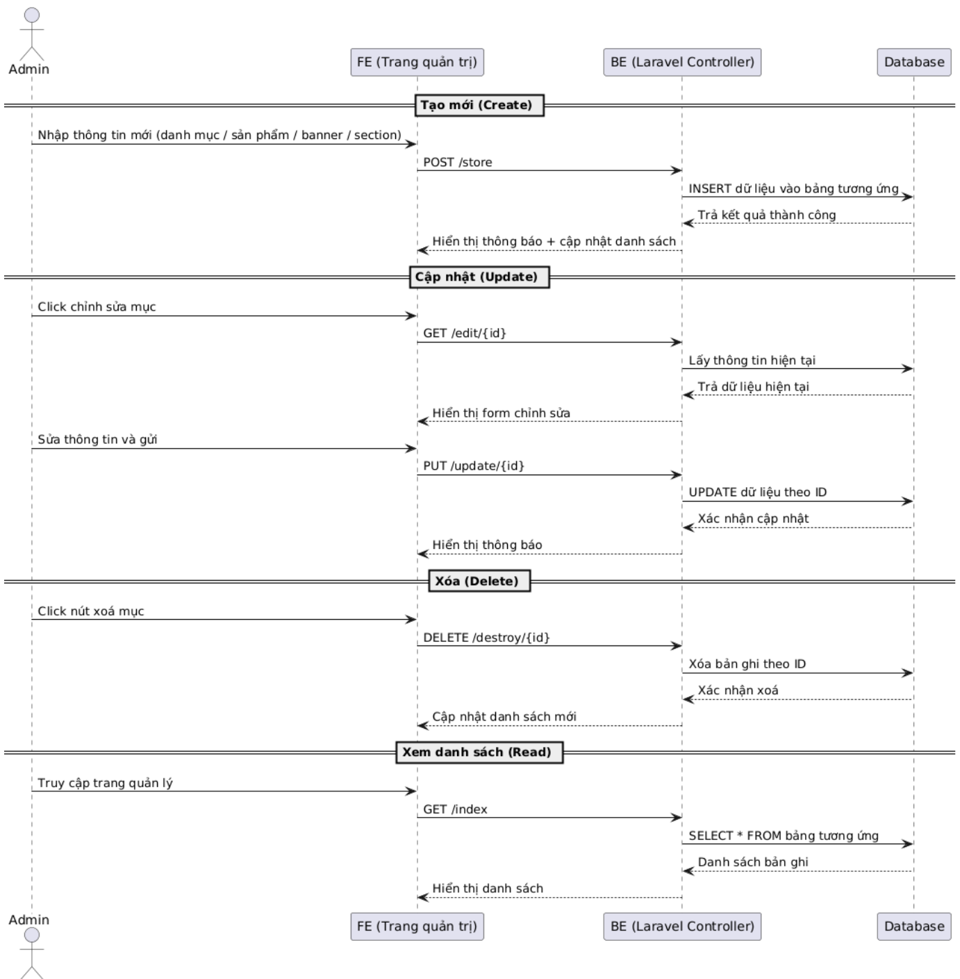
Hình 13 Sơ đồ tuần tự CRUD
