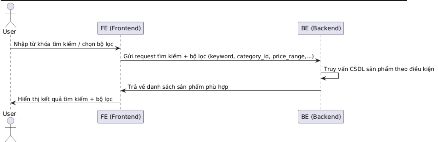
Hình 8 Sơ đồ tuần tự tìm kiếm sản phẩm
