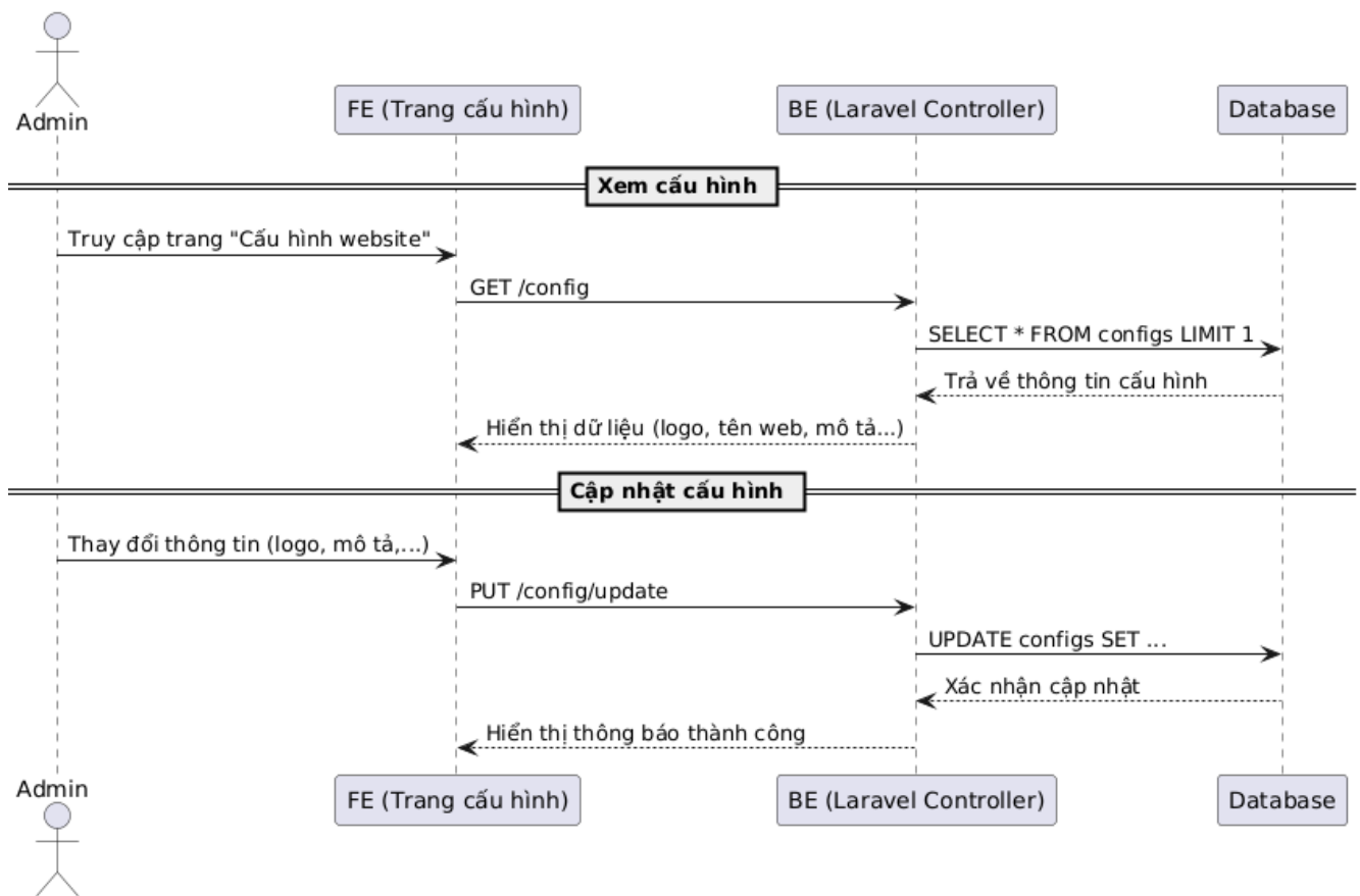
Hình 14 Sơ đồ tuần tự cấu hình website
