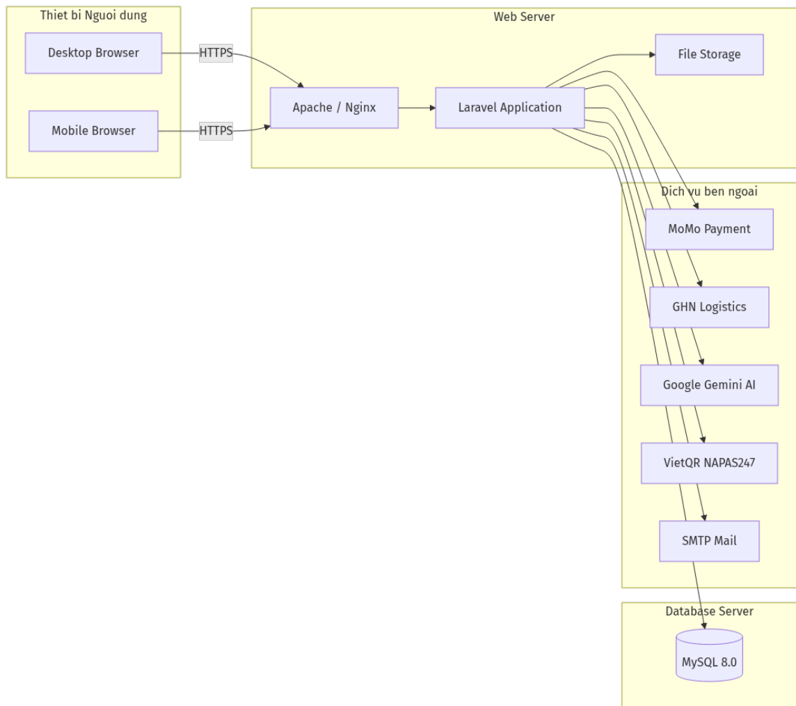
Hình 15: Sơ đồ triển khai hệ thống
