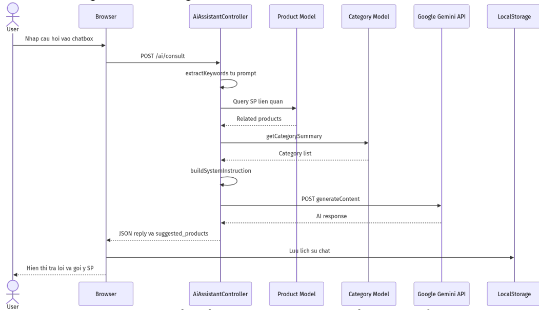
Hình 8: Sơ đồ tuần tự - Trợ lý AI tư vấn sản phẩm
