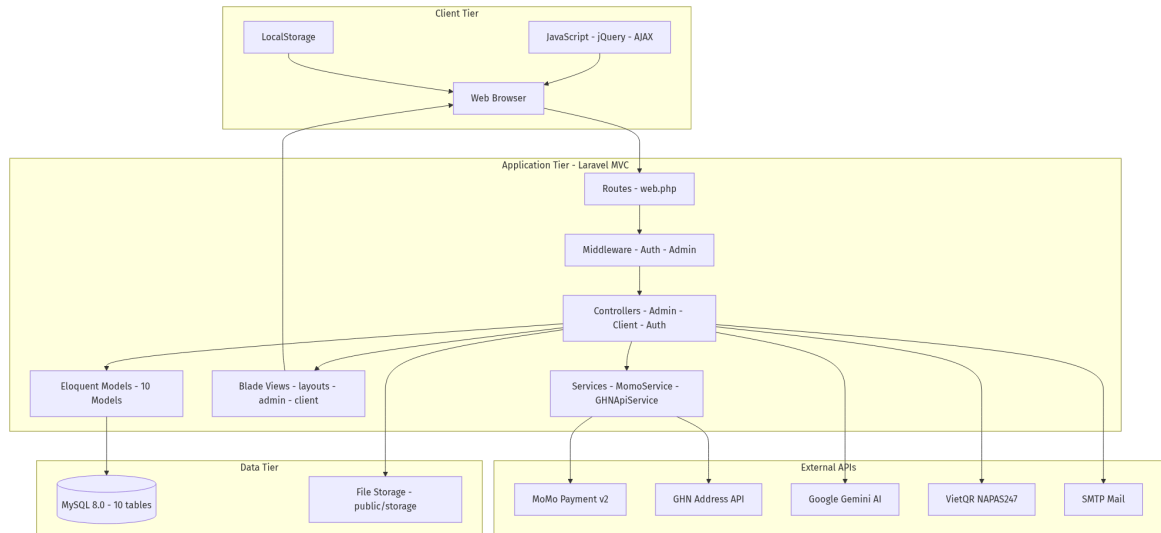
Hình 3: Kiến trúc tổng thể hệ thống
