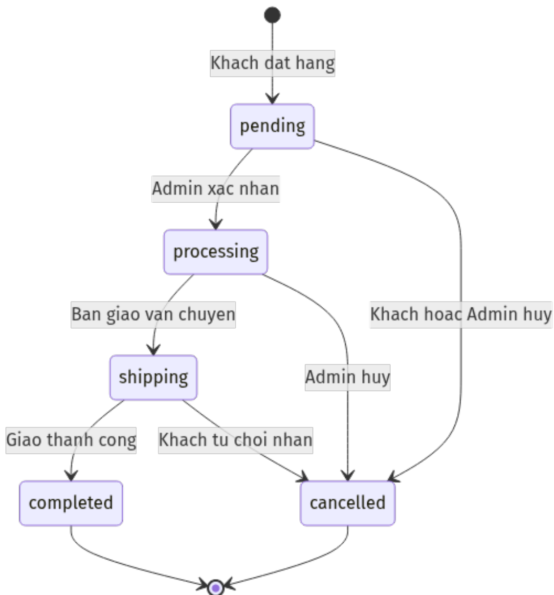
Hình 11: Sơ đồ trạng thái - Đơn hàng
