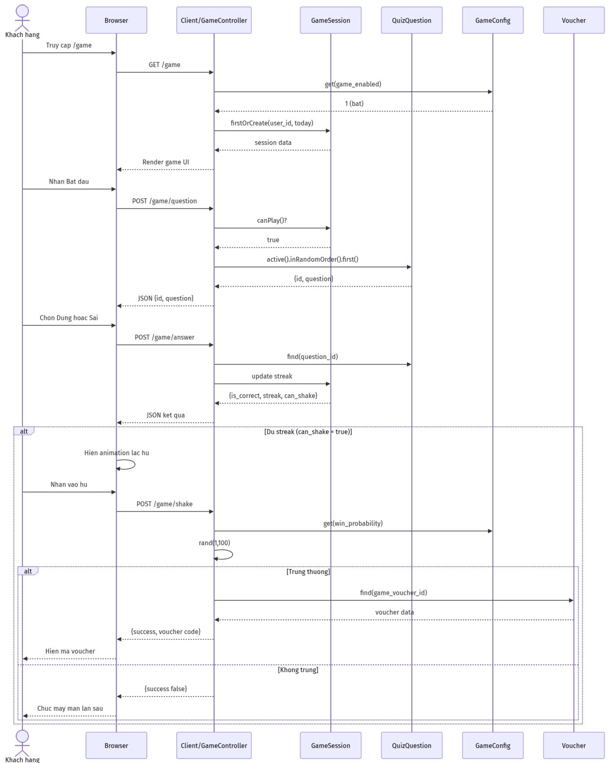
Hình 10: Sơ đồ tuần tự - Game Lắc Hũ
