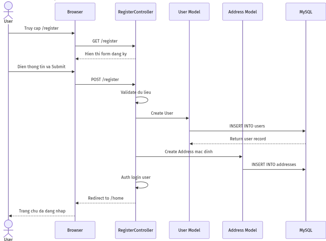
Hình 4: Sơ đồ tuần tự - Đăng ký tài khoản
