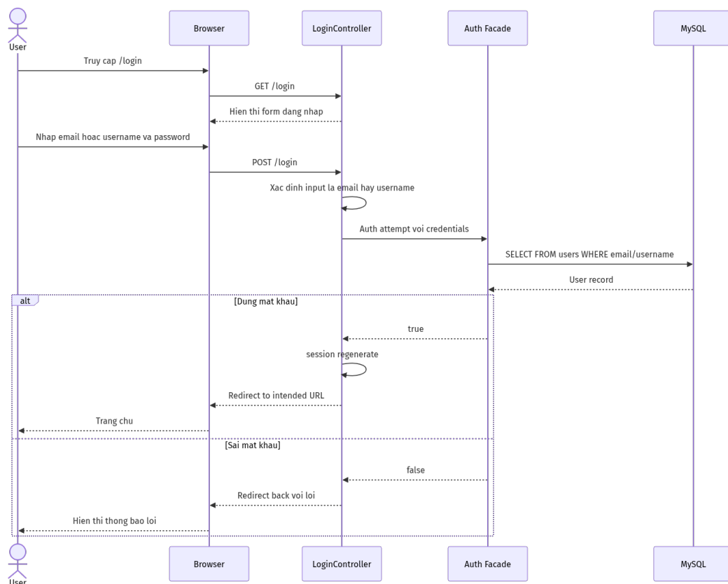
Hình 5: Sơ đồ tuần tự - Đăng nhập
