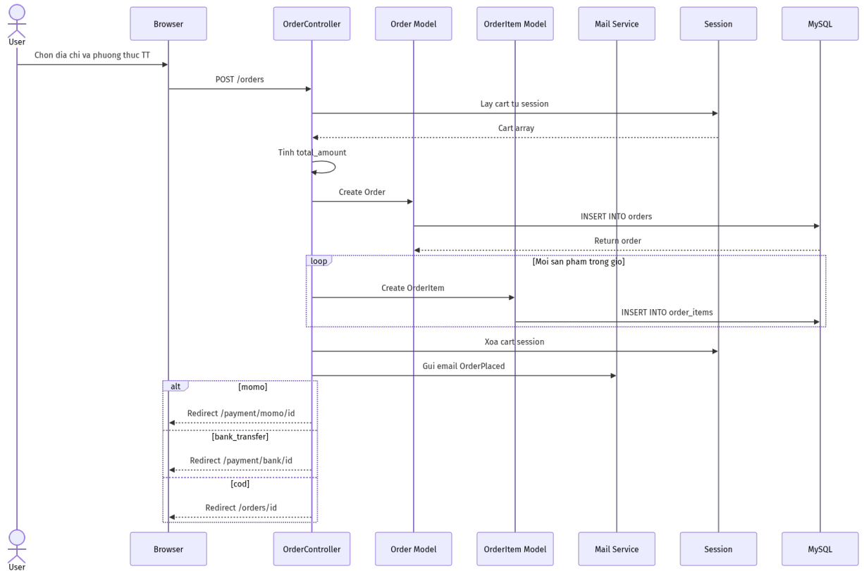
Hình 7: Sơ đồ tuần tự - Đặt hàng (Checkout)
