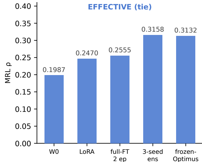
Real data (W ladder)
