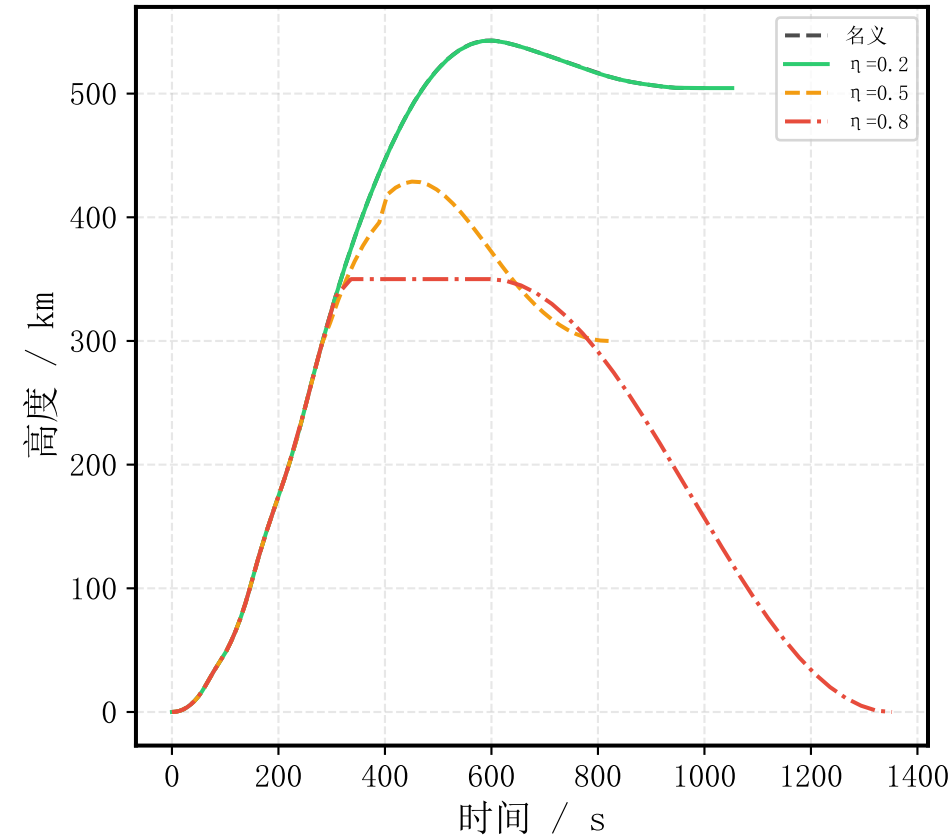
(e) F3: TVC卡滞
