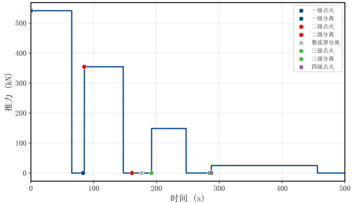
推力—时间曲线（动力上升段）
