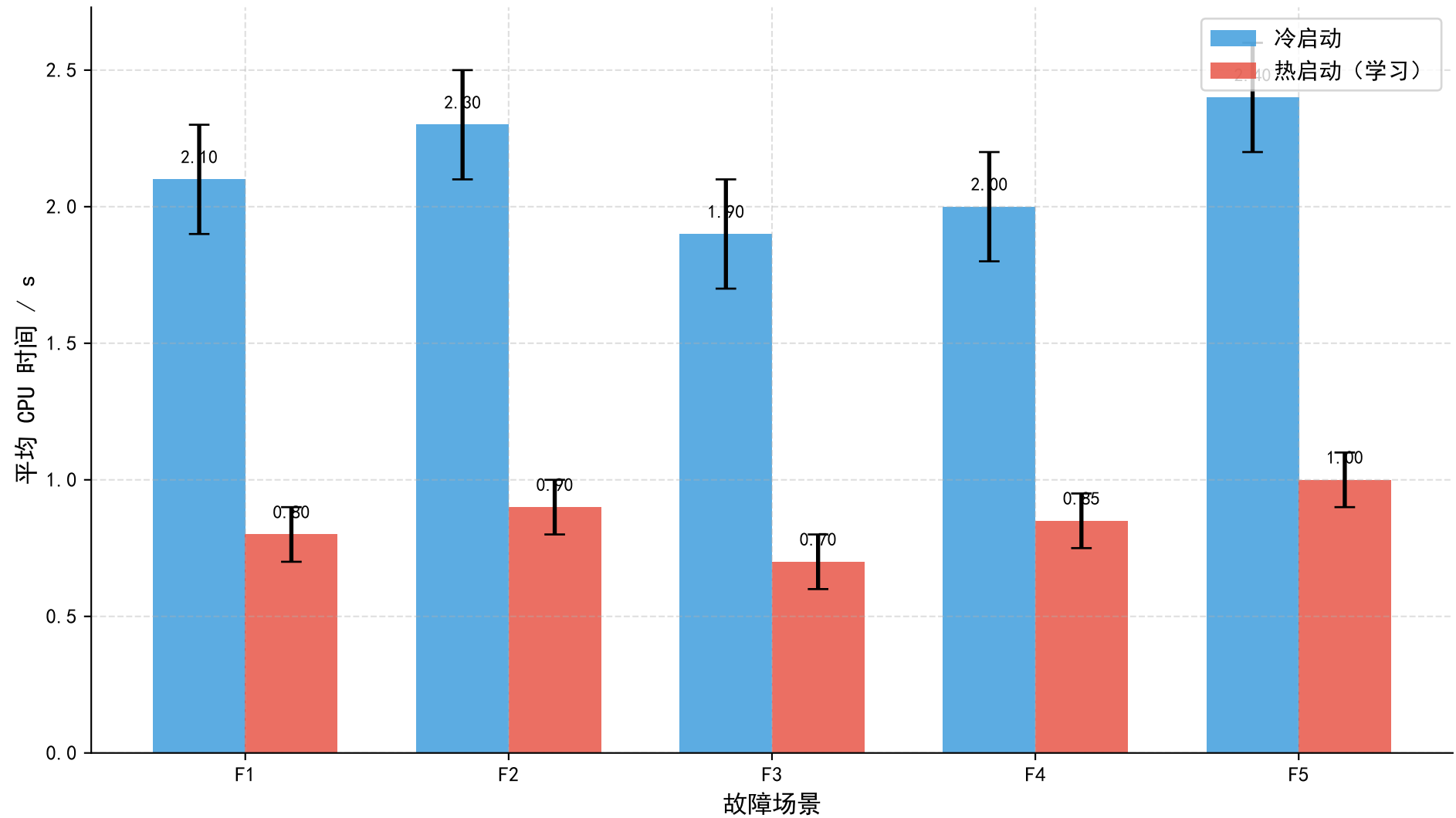
冷/热启动平均求解时间对比
