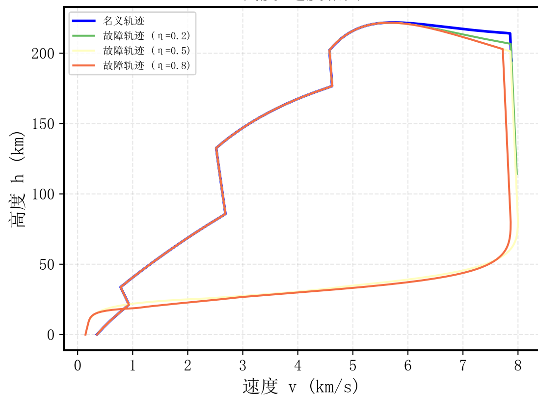
高度-速度相图
