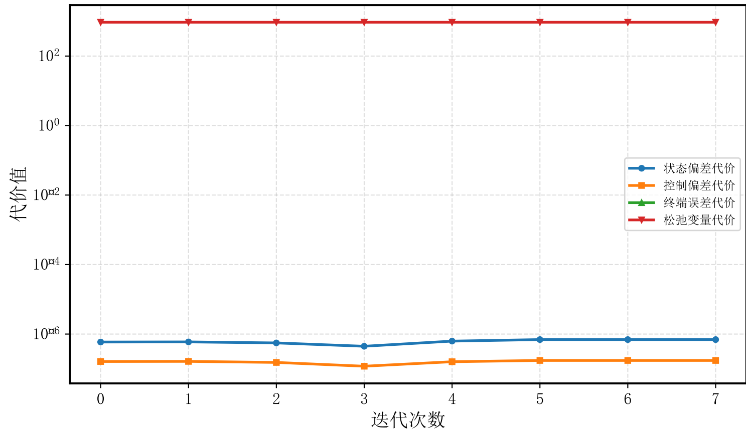
SCvx 收敛曲线：成本分解
