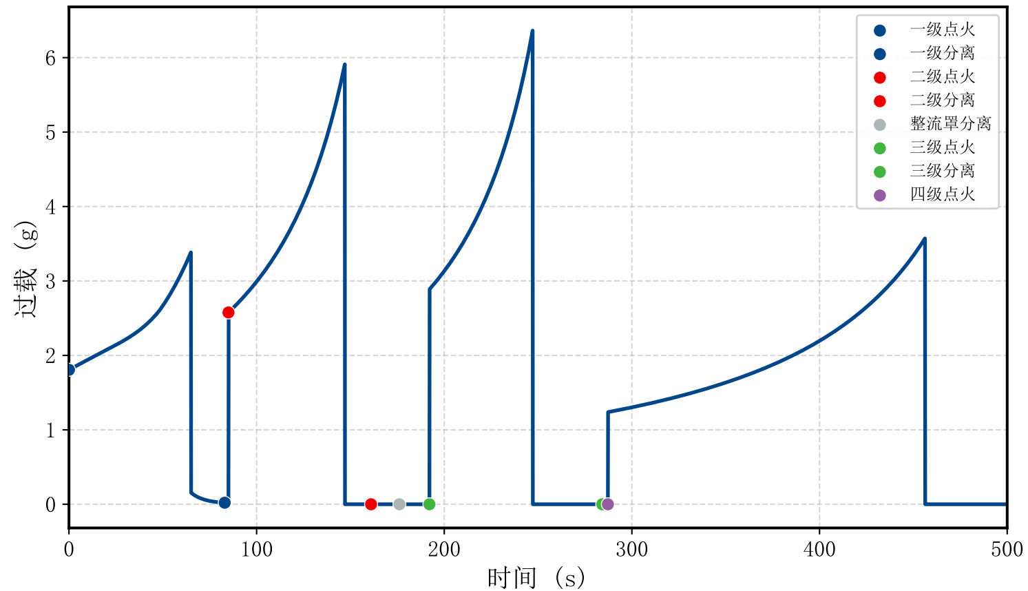
过载—时间曲线（动力上升段）
