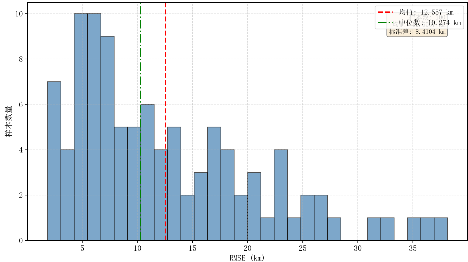
高度预测RMSE分布直方图
