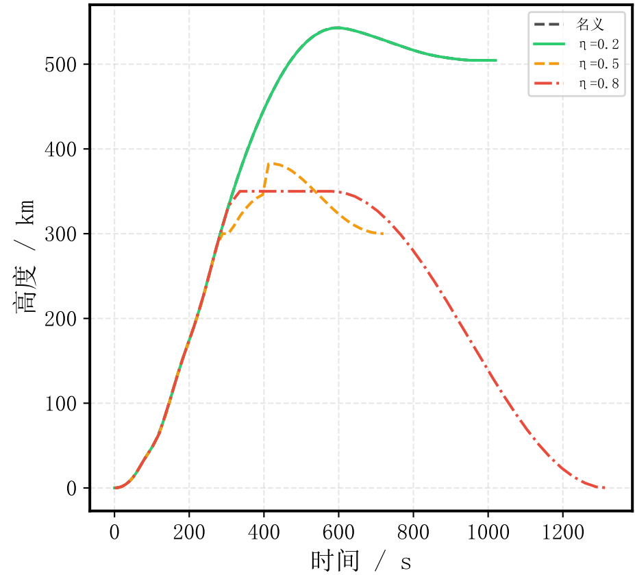
(d) F2: TVC速率限制
