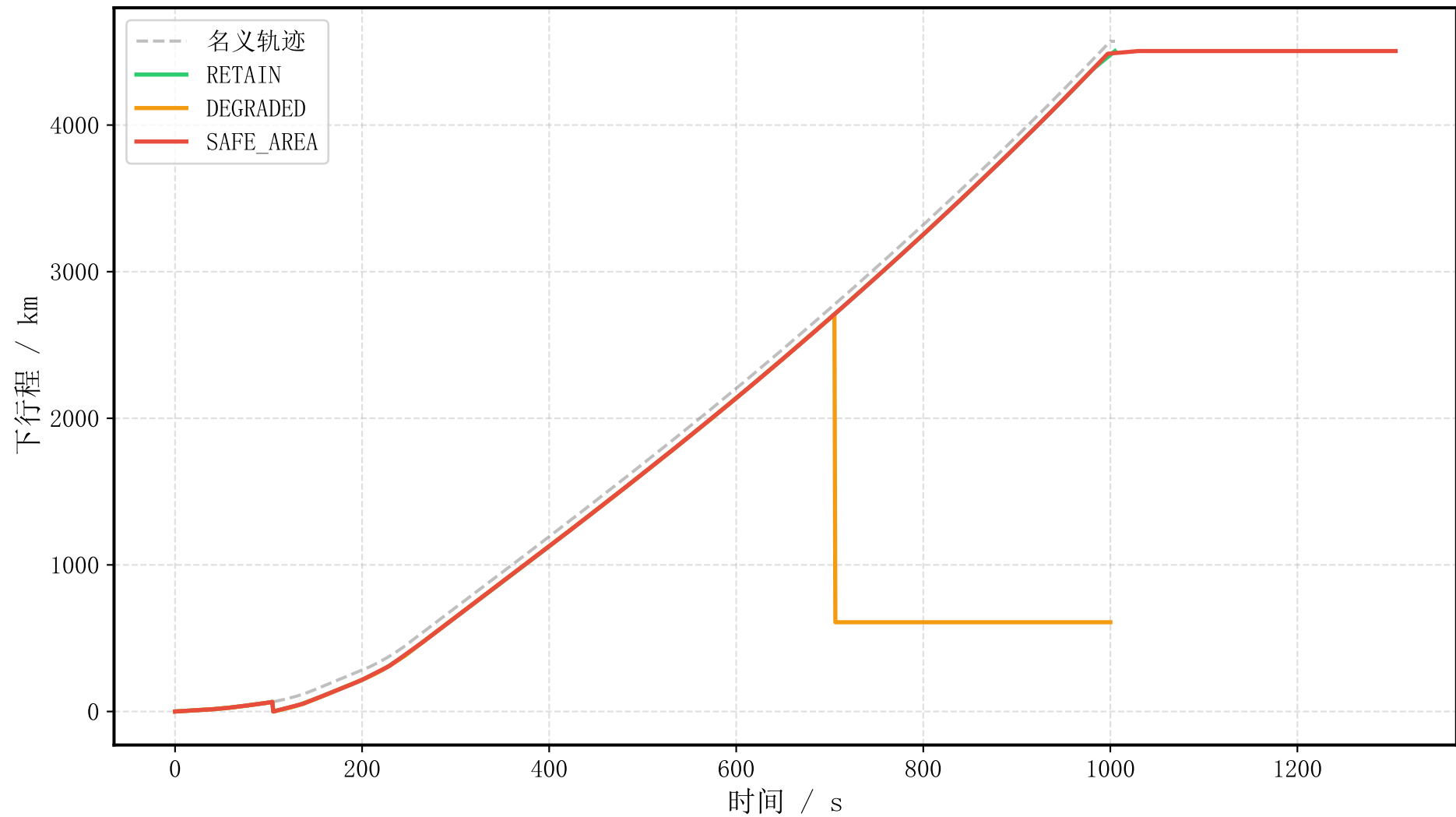
三任务域轨迹对比：下行程 ( F_{l\_thrust\_deg15} , \eta=0.8 )
