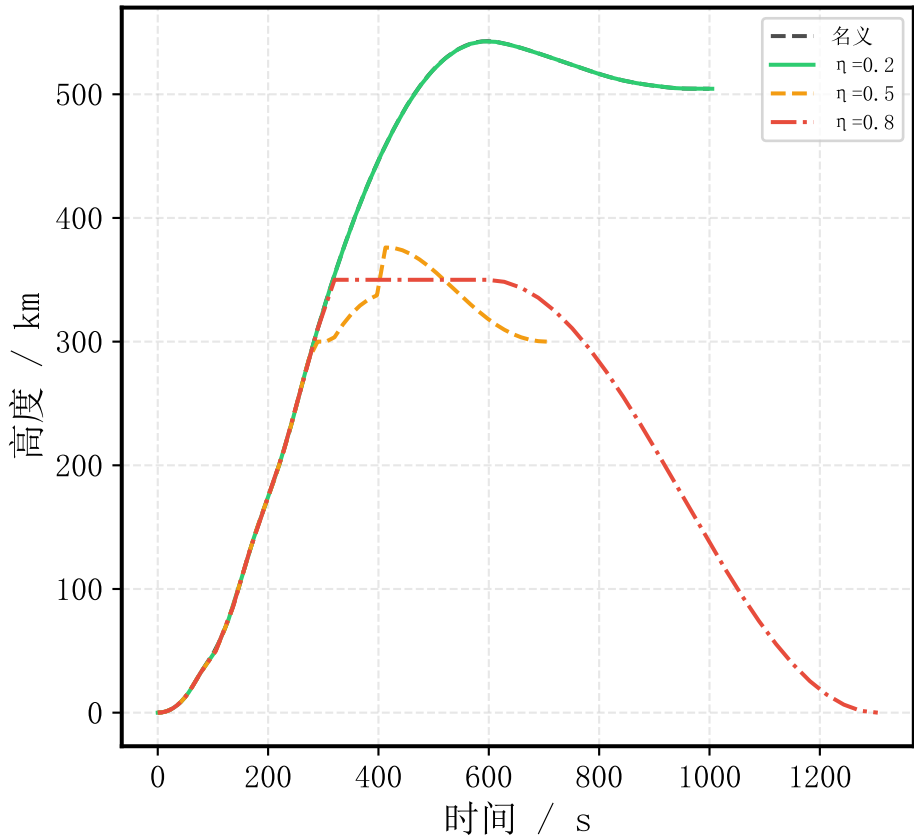
(c) F1: 推力降级
