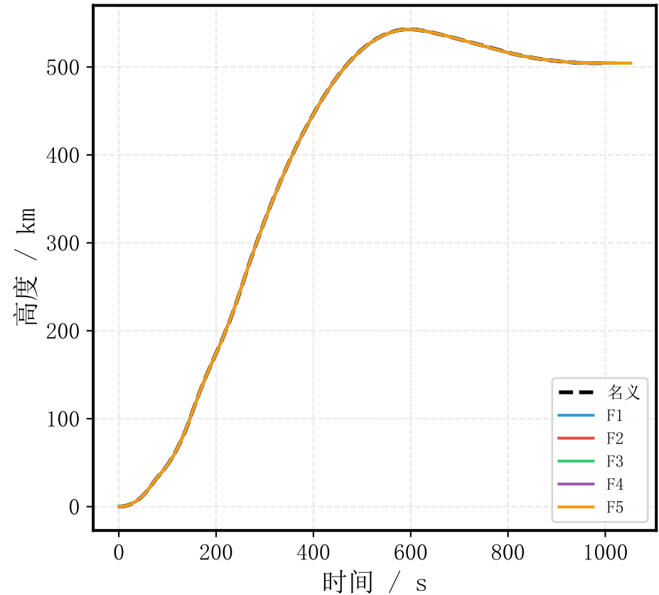
(a) 高度响应
