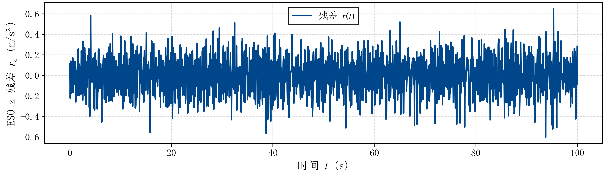
ES0 z 轴残差波形（名义工况）
