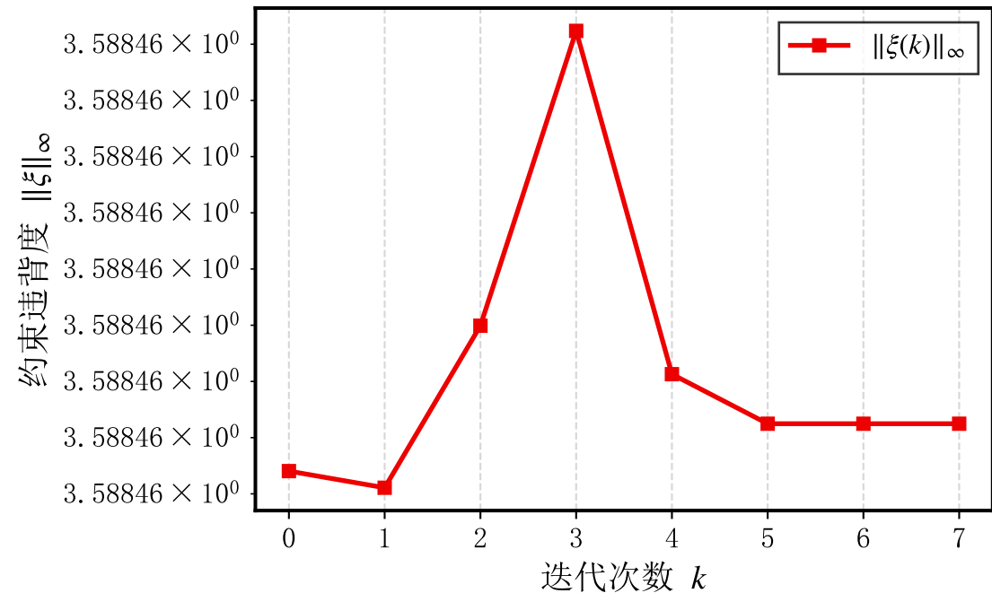
SCvx 收敛曲线：约束可行性
