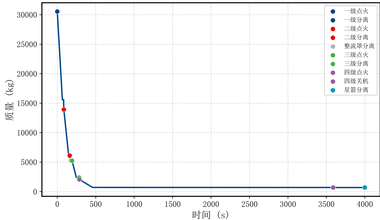
质量—时间曲线
