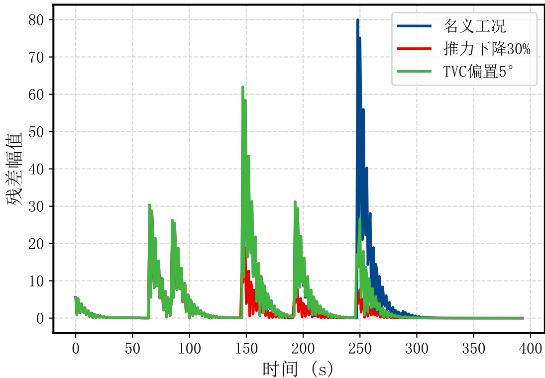
ESO残差对比
