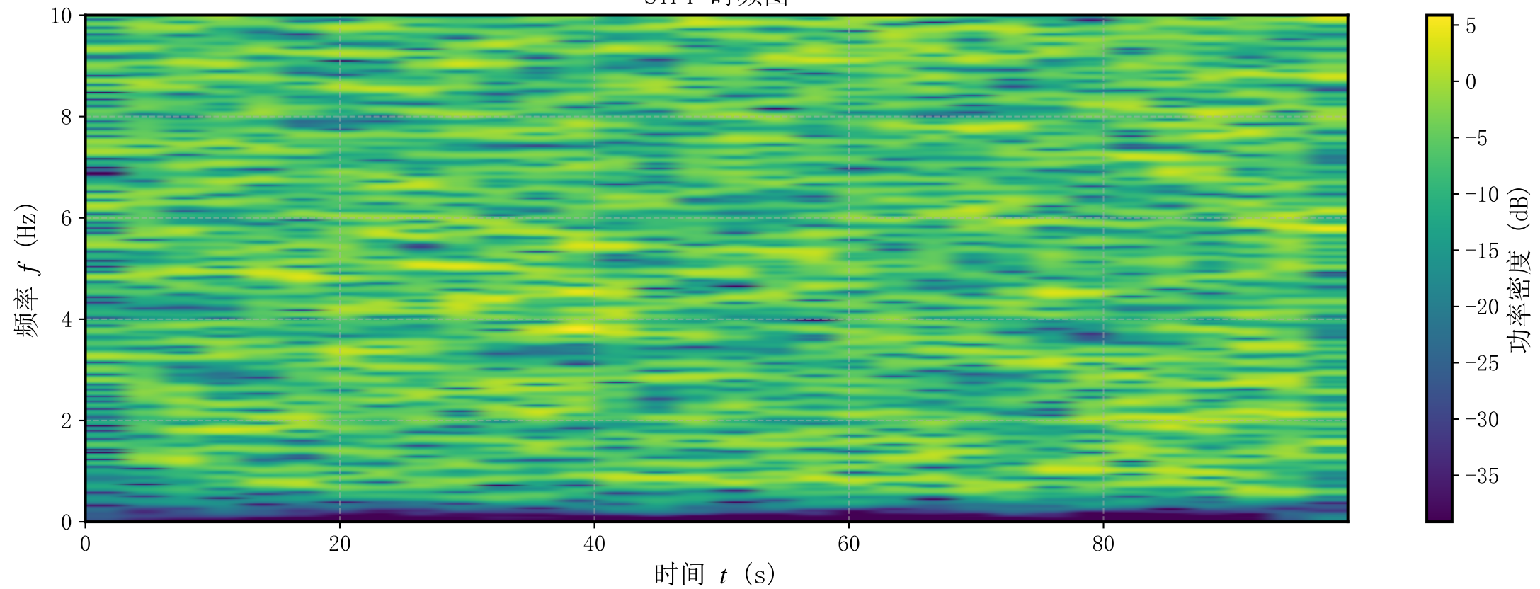
STFT 时频图
