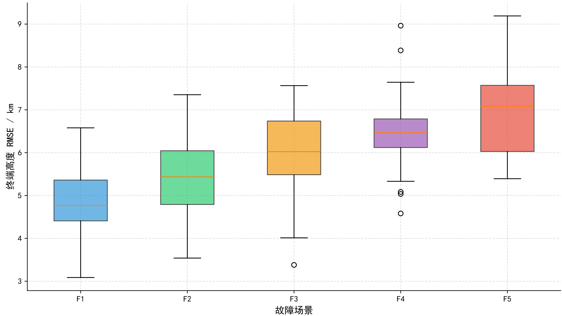
不同故障下终端高度 RMSE 分布
