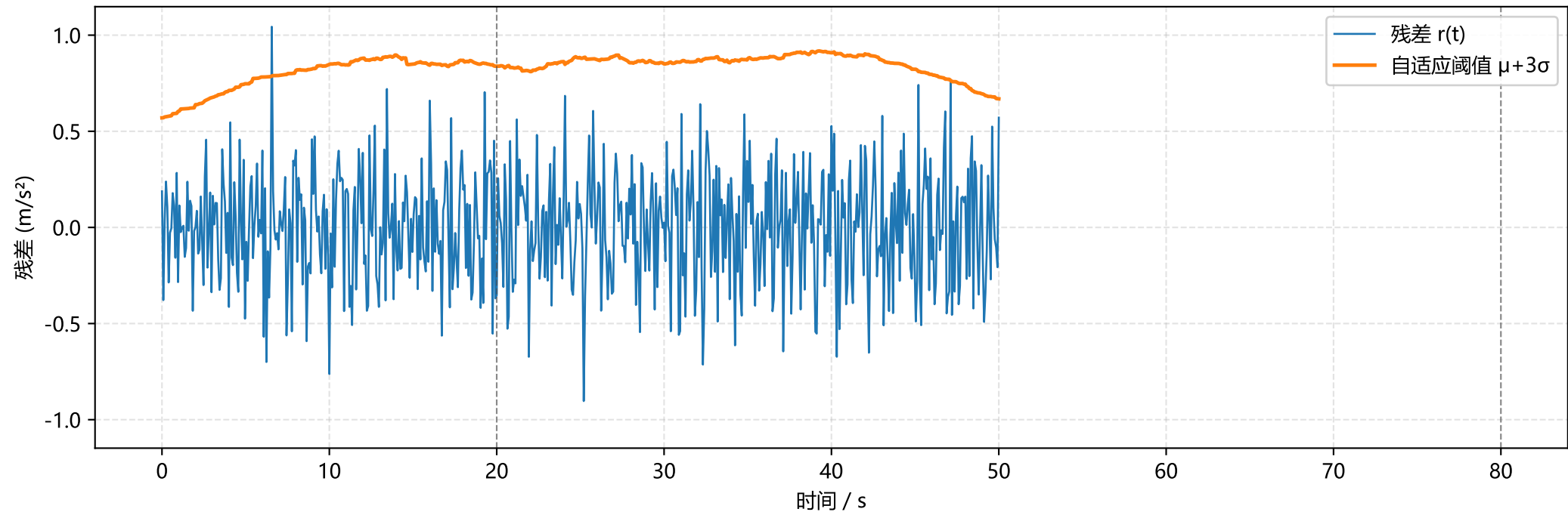
图3-8 残差序列与自适应阈值对比
