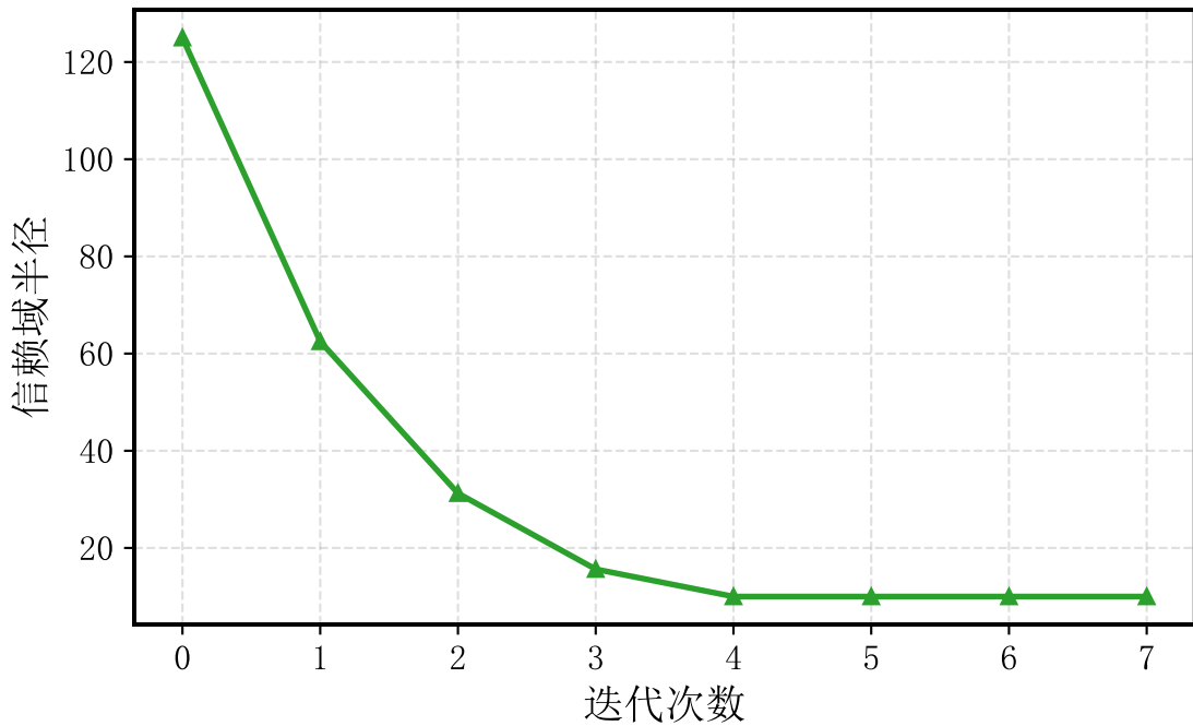
SCvx 收敛曲线：信赖域
