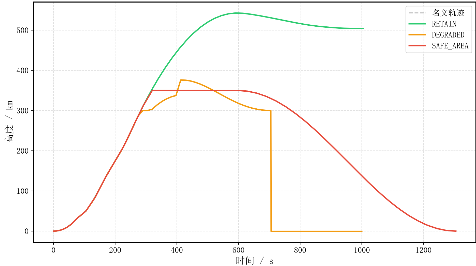
三任务域轨迹对比：高度 (F1_thrust_deg15, \eta=0.8 )
