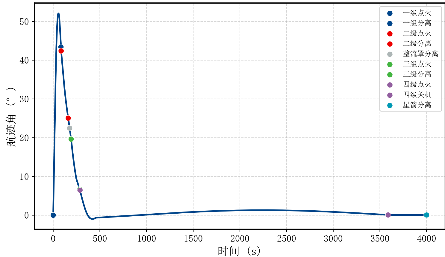
航迹角—时间曲线
