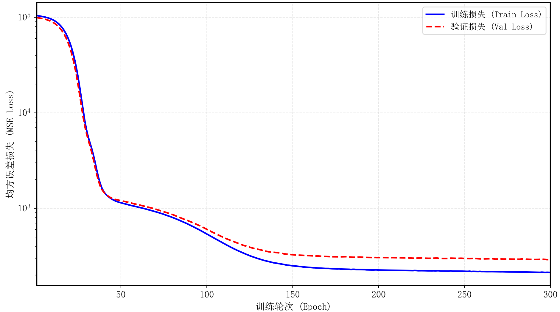
学习热启动模型训练曲线
