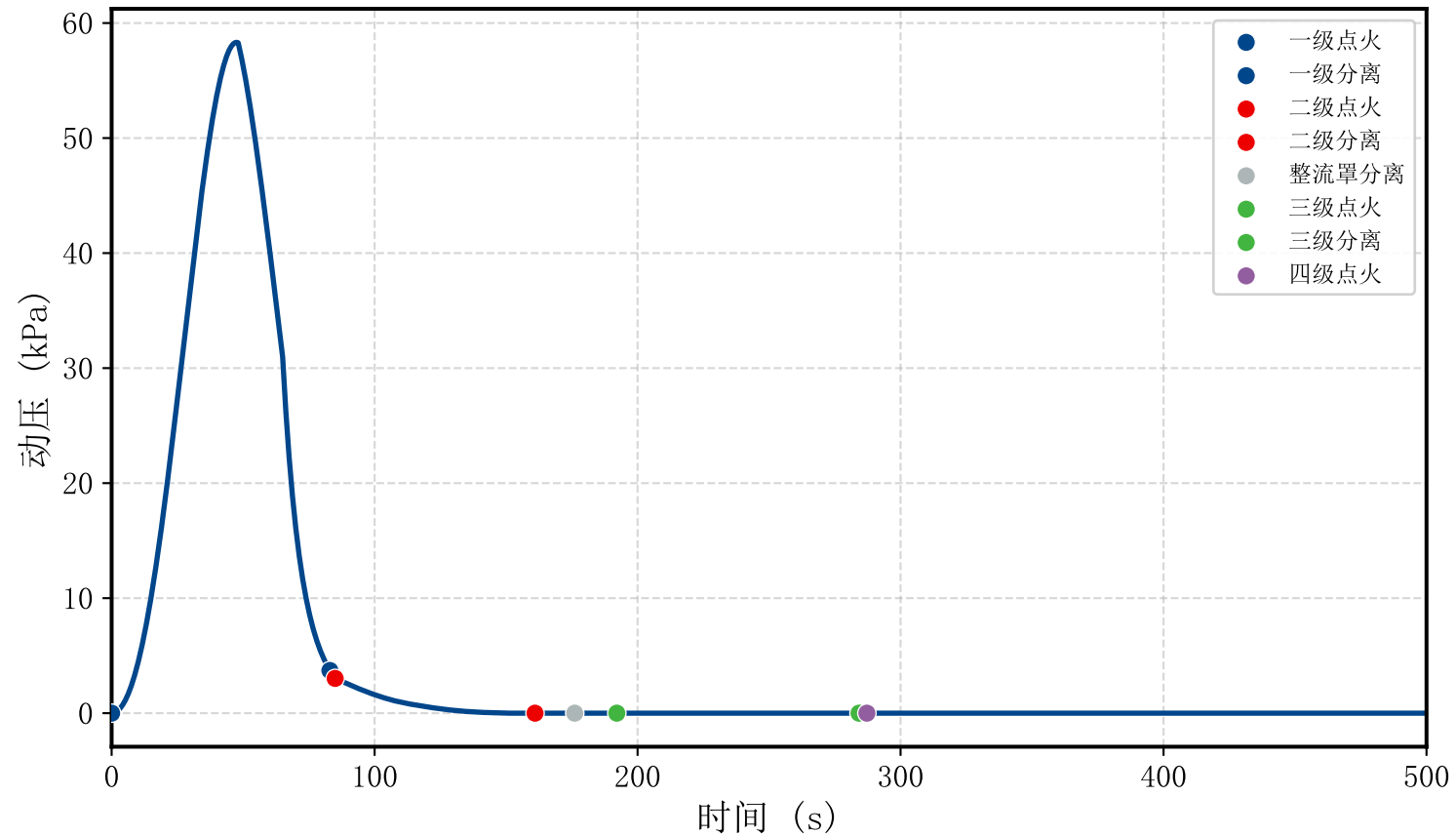
动压—时间曲线（动力上升段）
