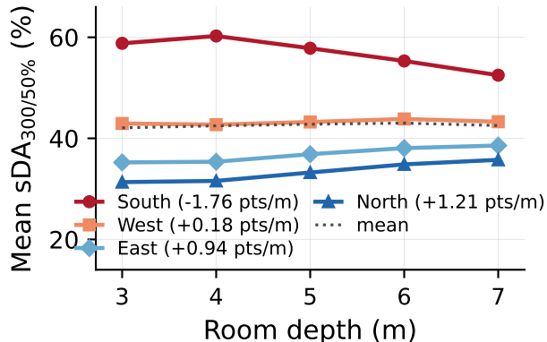
(d) Room depth, H/W = 0.0, by orientation
