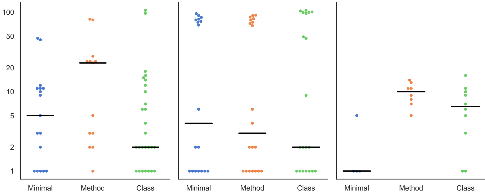
GPT-4o
