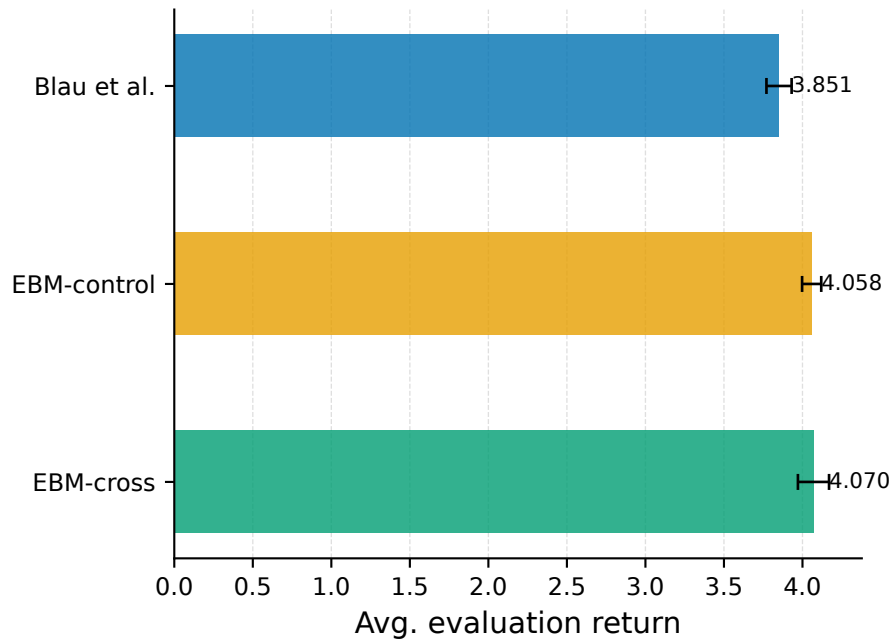
(b) Evaluation return
