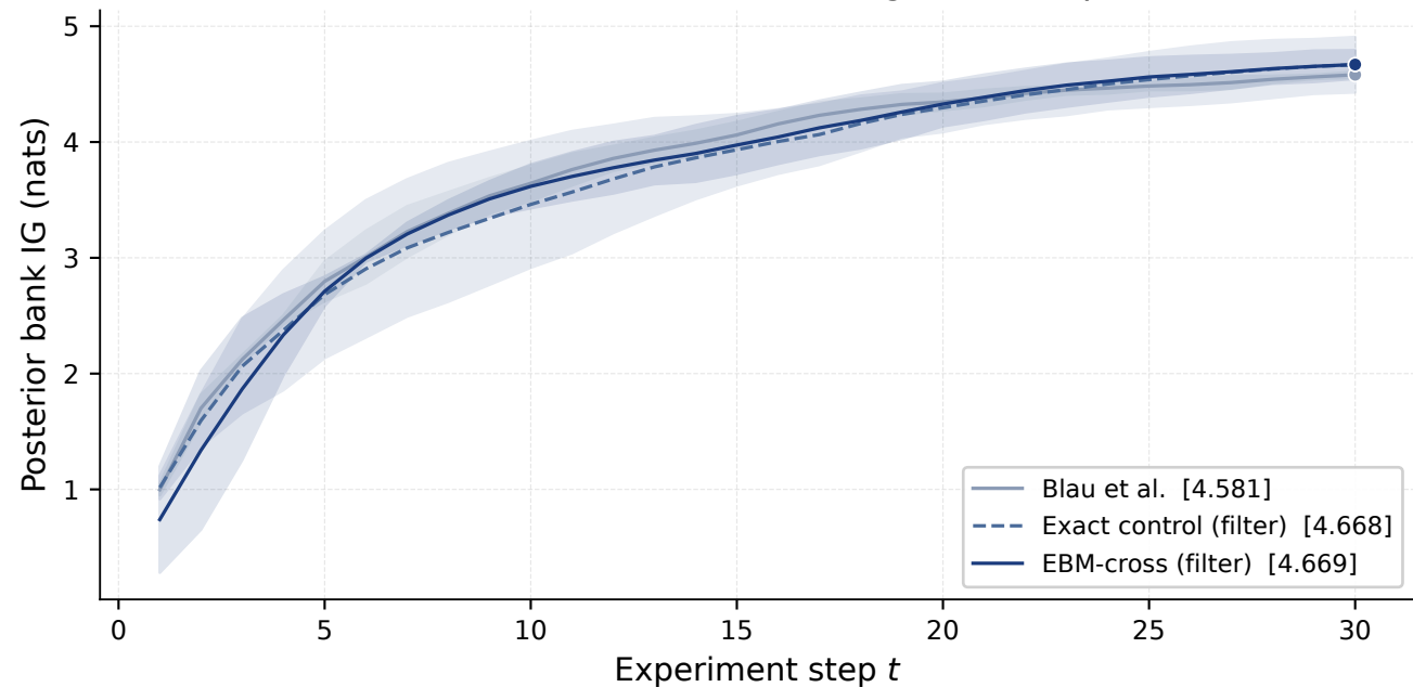
Posterior bank information gain vs. step
