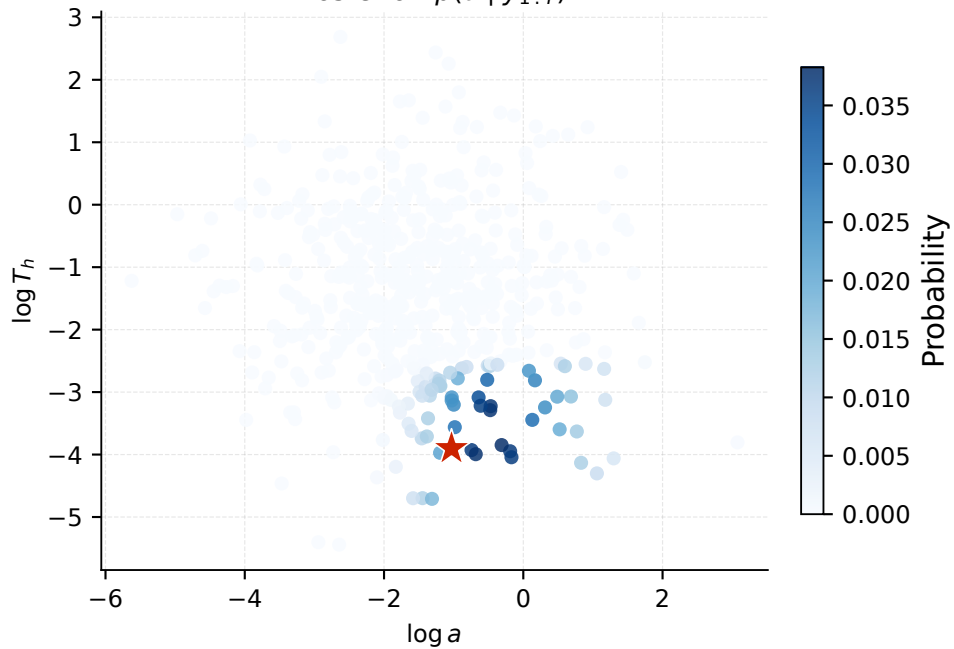
Posterior p(\theta | y_{1:T})
