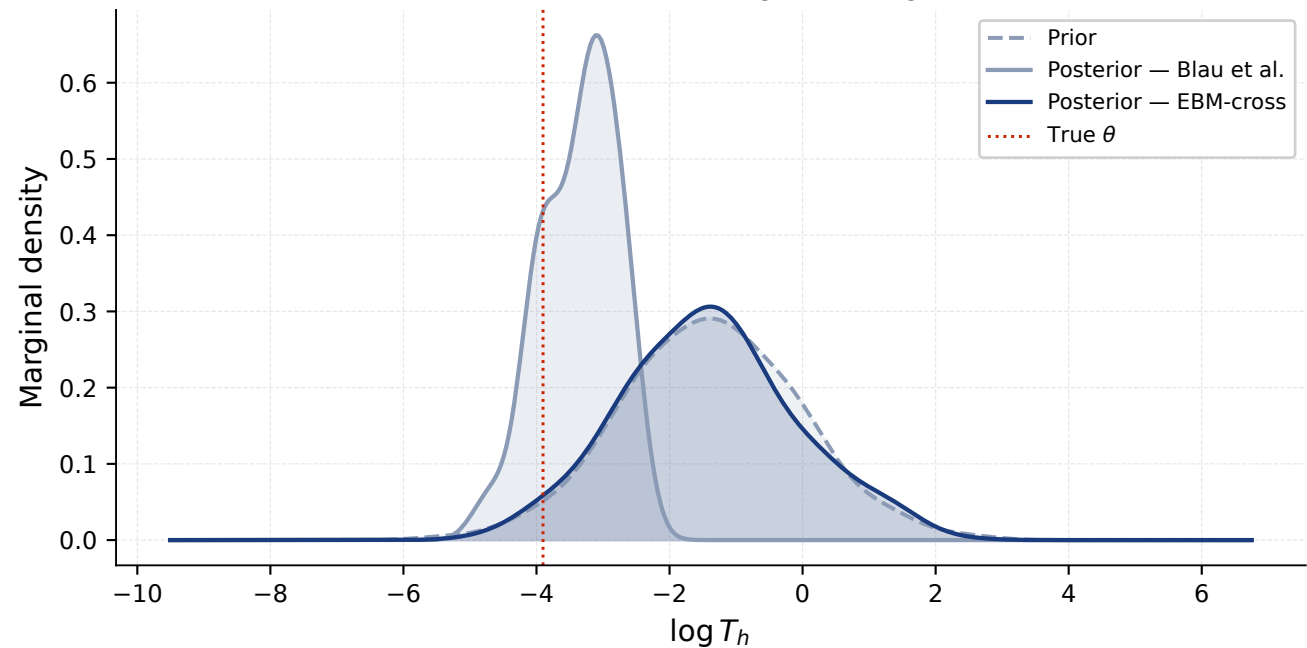
Prior vs Posterior marginals — \log T_h
